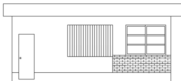
東立面図
