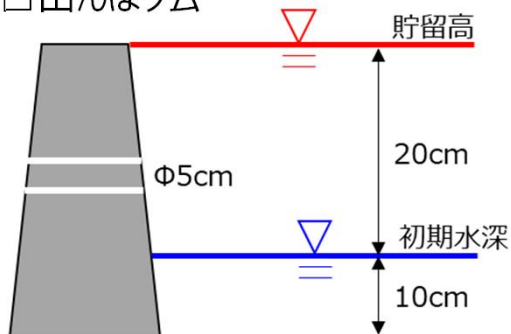
図 田んぼダムモデル図
