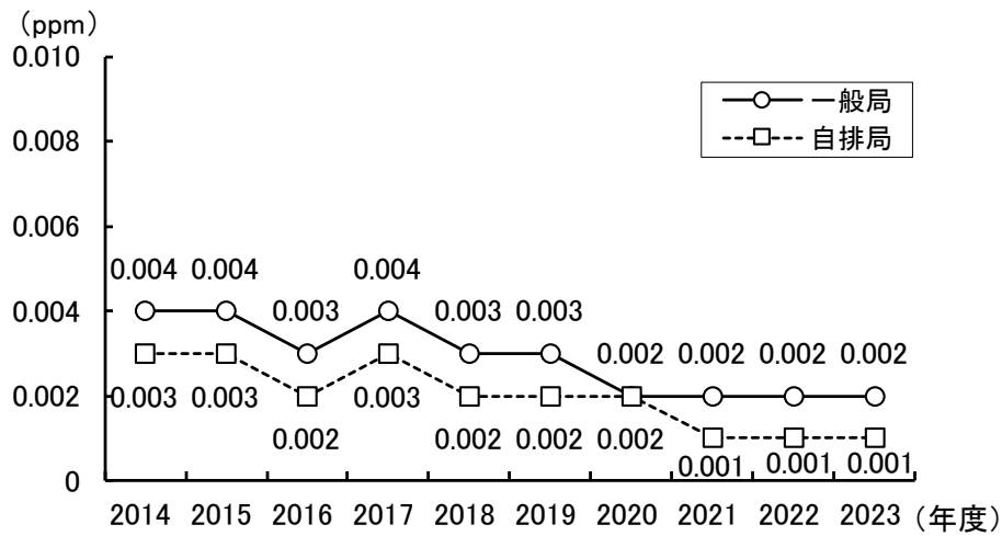
図5-1 二酸化硫黄の年平均濃度の推移
