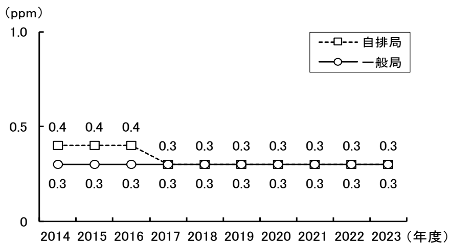
図5-2 一酸化炭素の年平均濃度の推移
