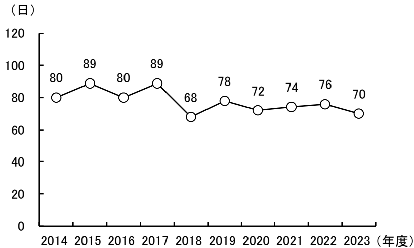
図4-1 光化学オキシダントの昼間の濃度が環境基準値を超えた日数の推移
