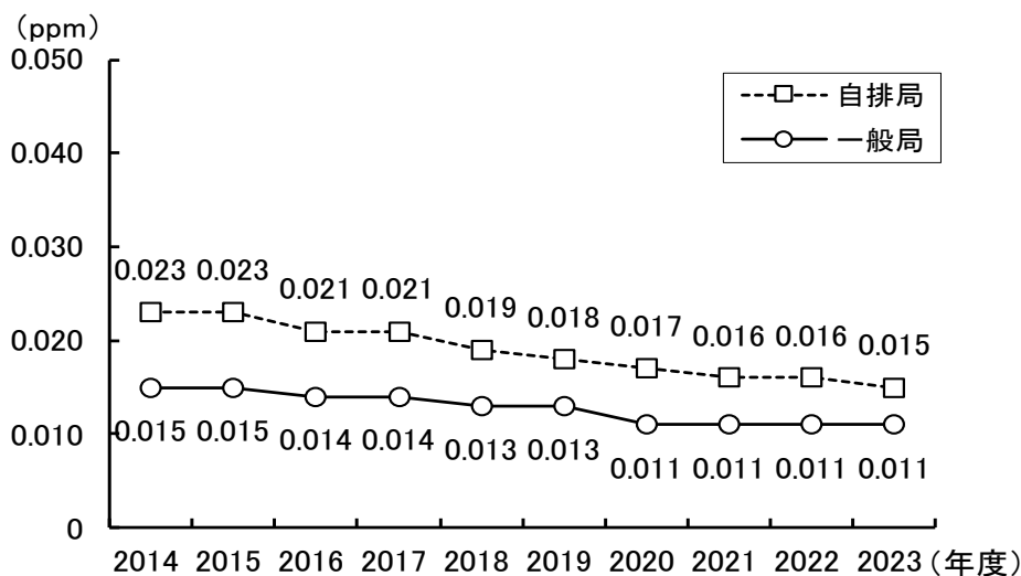
図 1-2 二酸化窒素の年平均濃度の推移
