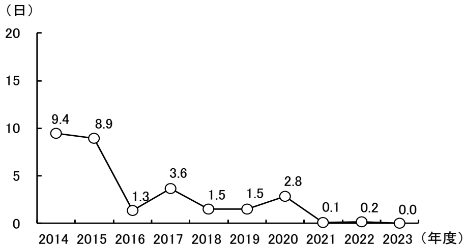
図3-3 微小粒子状物質の日平均値が 35\mu\text{g}/\text{m}^3 を超えた日数の平均の推移
