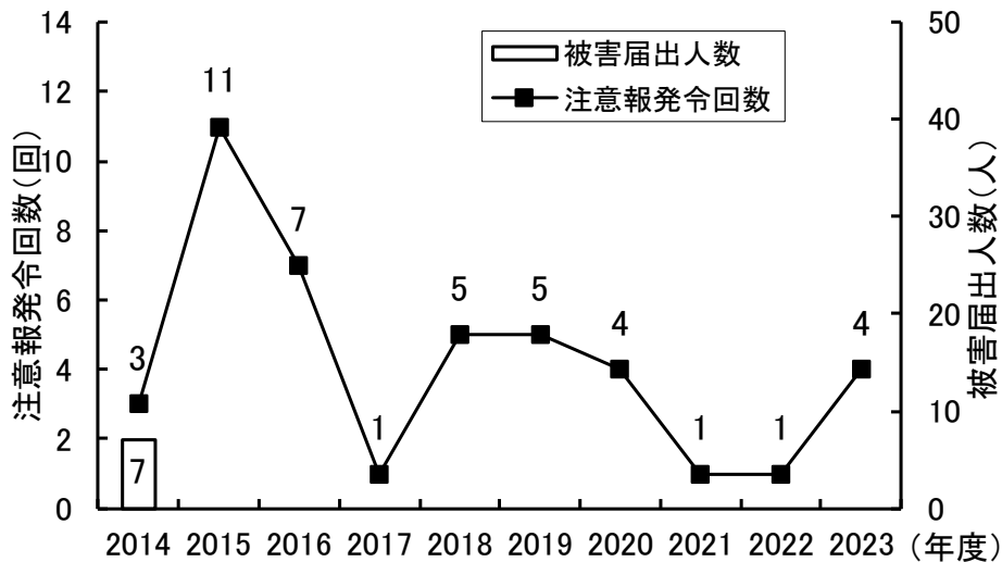
図4-2 光化学スモッグ注意報の発令回数と被害届出人数の推移
