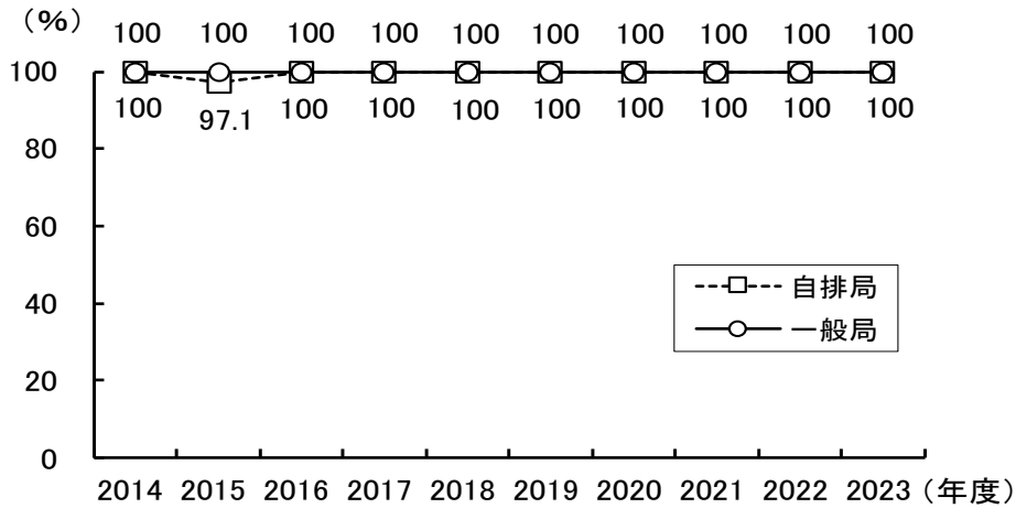
図2-1 浮遊粒子状物質の長期的評価による環境基準達成率の推移
