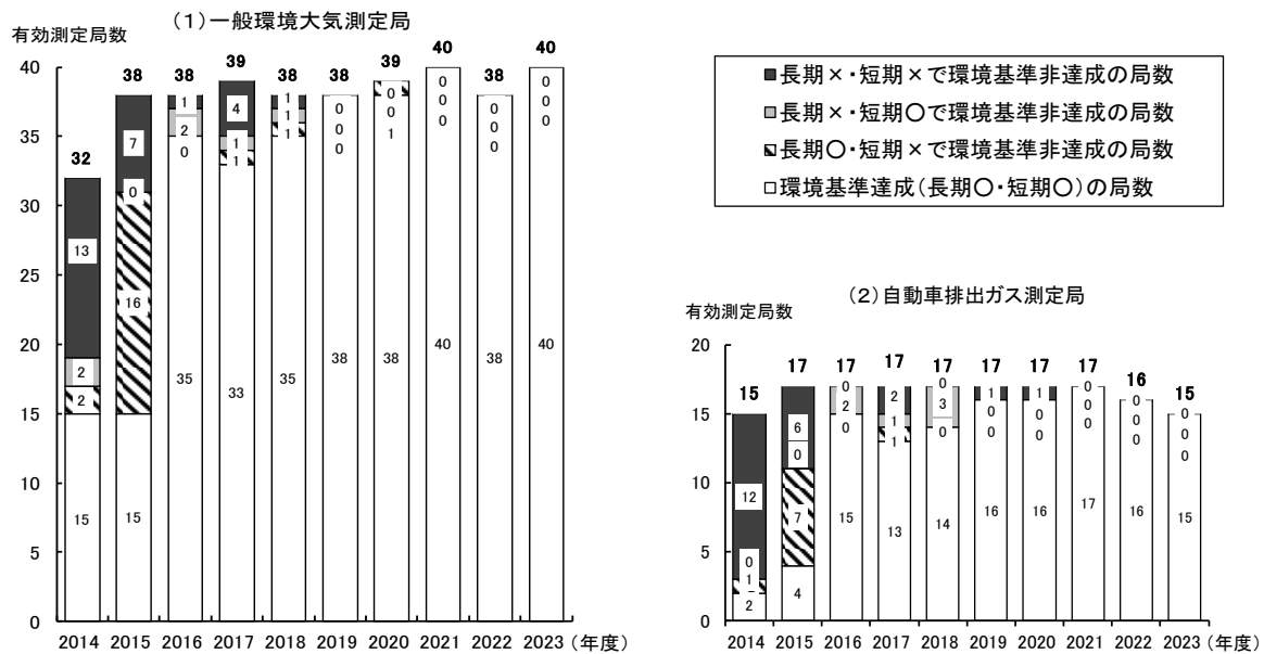
図3-1 微小粒子状物質の環境基準達成状況の推移
