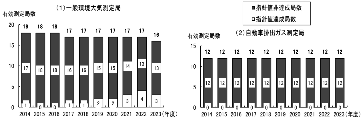
図4-4 非メタン炭化水素の指針値達成状況の推移
