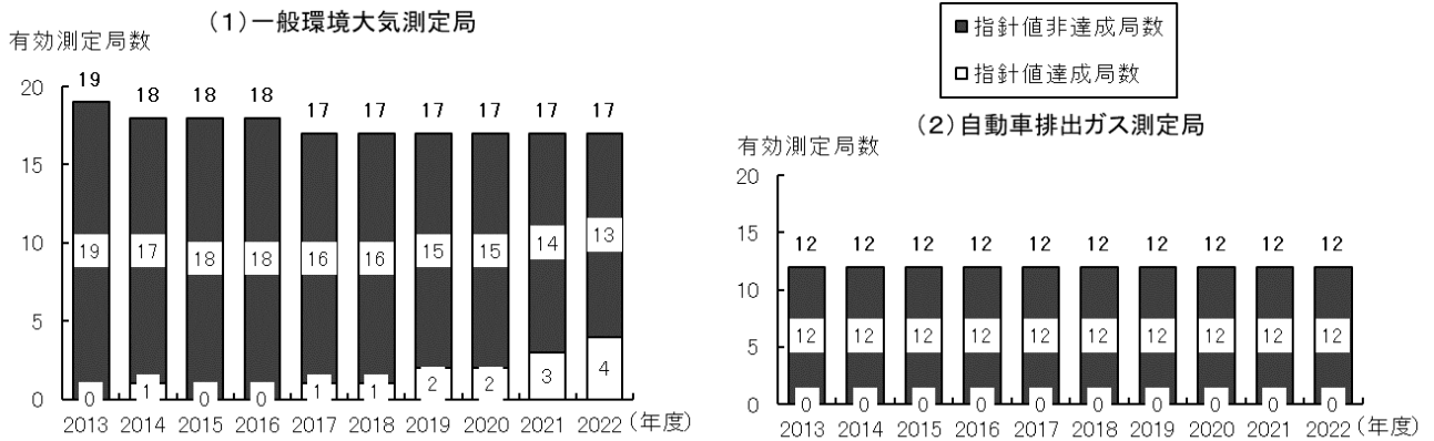
図4-4 非メタン炭化水素の指針値達成状況の推移
