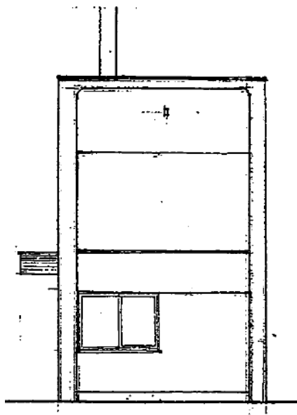
西立面図
