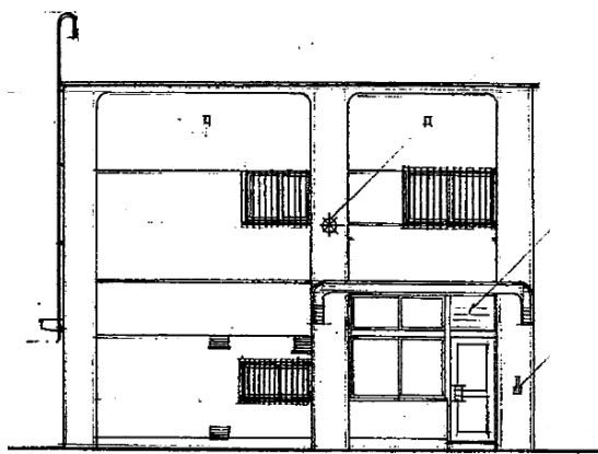
北立面図
