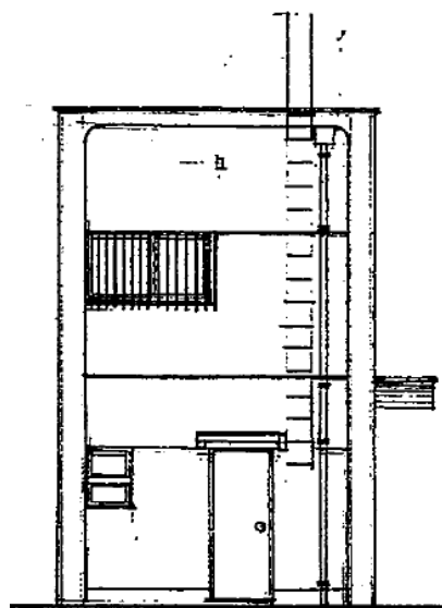
東立面図
