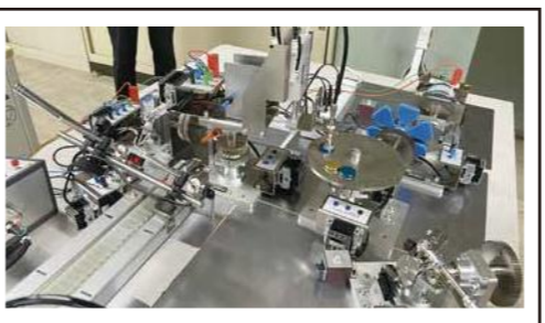
メカトロニクス技術実習システム ロボットやベルトコンベアなどを組み合わせて、メカトロニクスの基礎から応用まで幅広く学べる装置です。
