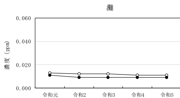
第 10. 1. 1. 1-11 図(5) 窒素酸化物の年平均値の経年変化
