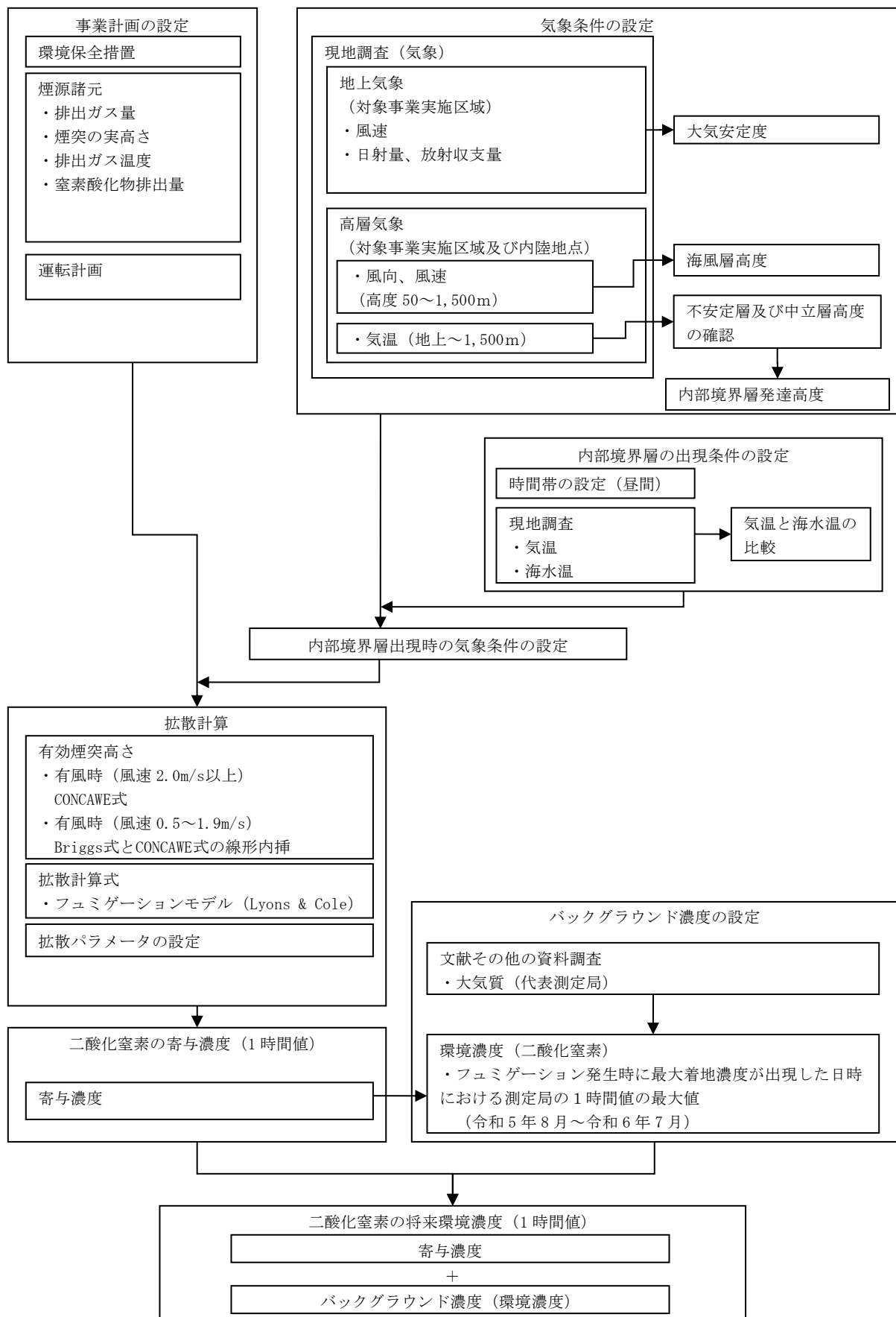
第 10. 1. 1. 1-42 図 内部境界層によるフミゲーション発生時の予測手順
