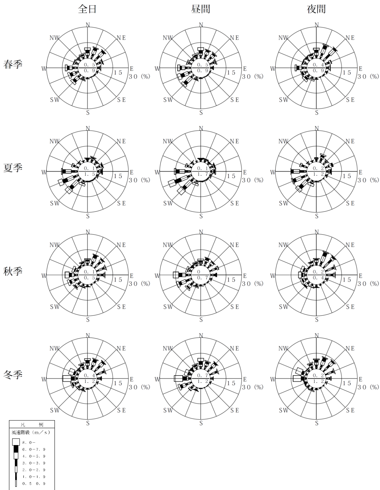
第 10. 1. 1. 1-4 図(2) 風速階級別風配図 (上層・季節別)
