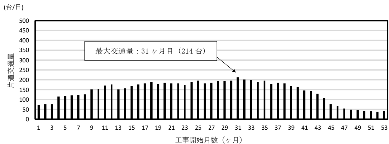
第 10.1.1.1-25 図 工事関係車両の月別交通量
