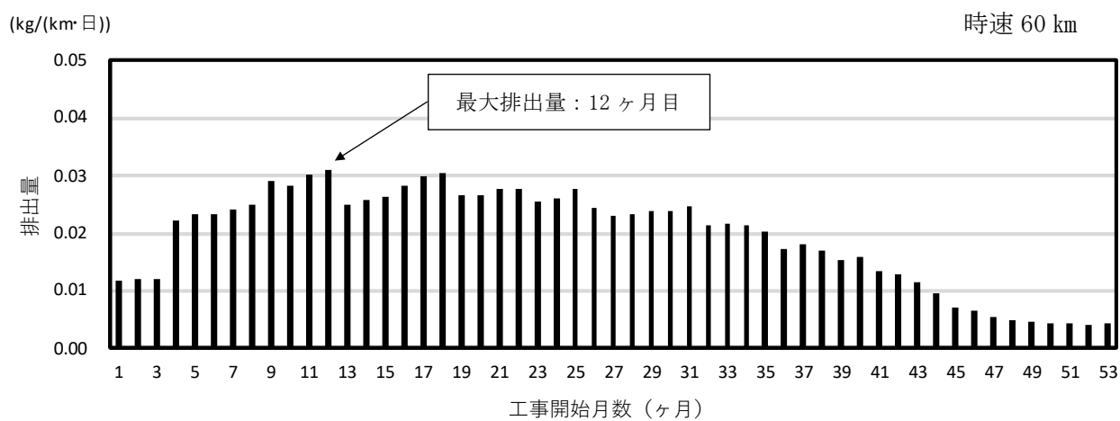
第 10. 1. 1. 1-23 図(2) 工事関係車両による浮遊粒子状物質の月別日平均排出量
