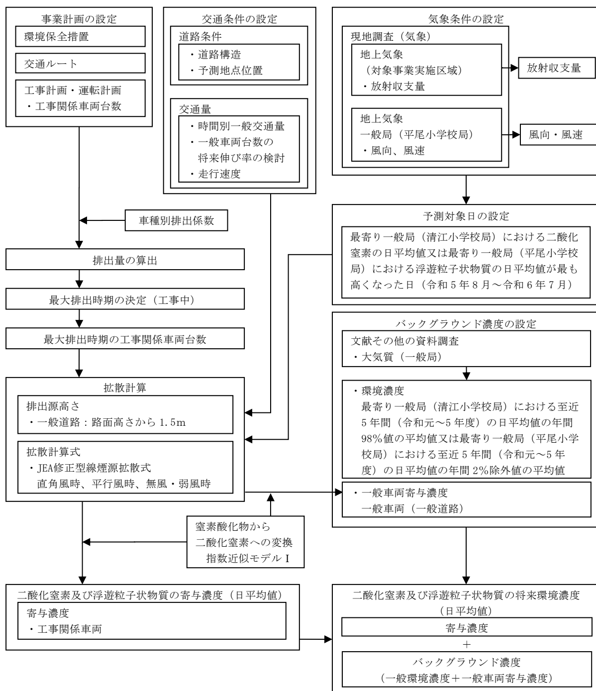
第 10.1.1.1-24 図 工事用資材等の搬出入による二酸化窒素及び浮遊粒子状物質の予測手順
