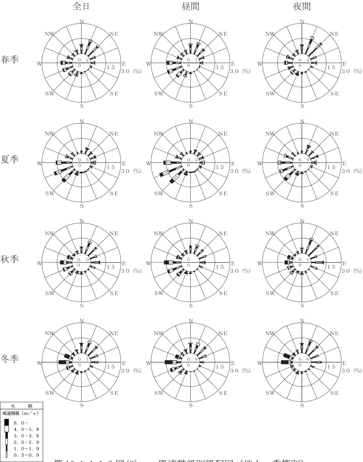
第 10.1.1.1-3 図(2) 風速階級別風配図（地上・季節別）
