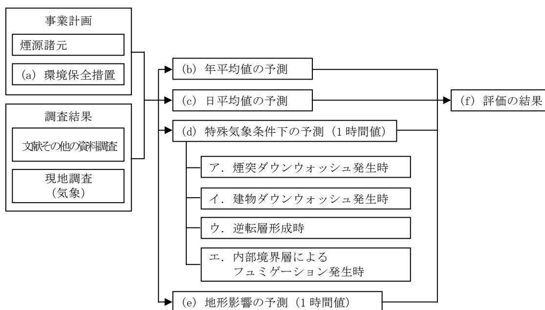
第10.1.1.1-29 図 施設の稼働（排ガス）に係る予測の概念図
