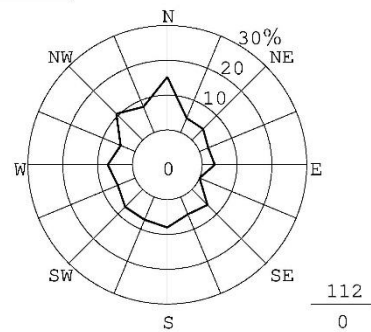
第 10.1.1.1-5 図(4) 高度別風配図（高層・秋季）（対象事業実施区域）
