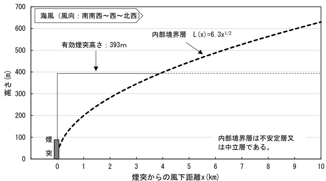
第 10. 1. 1. 1-43 図(1) 内部境界層によるフュミゲーション発生時のモデル化図 (定常運転時)
