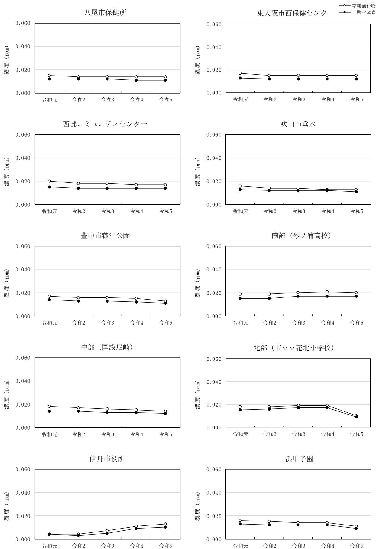
第 10. 1. 1. 1-11 図(4) 室素酸化物の年平均値の経年変化
