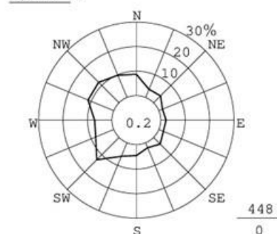
第 10.1.1.1-5 図(1) 高度別風配図（高層・全季節）（対象事業実施区域）
