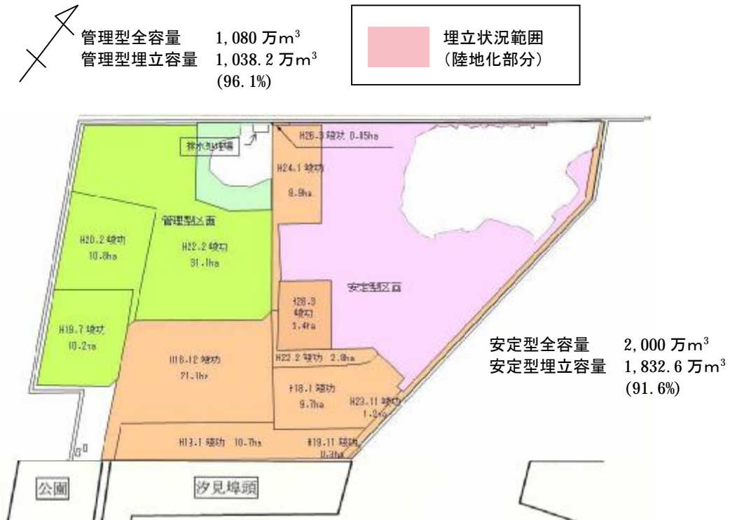
図 2-2-5 埋立の進捗状況(平成 27 年 3 月末現在)
