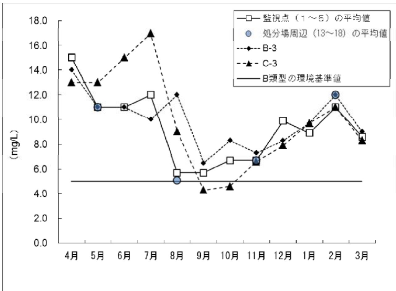
図 3-1-4 DO (上層) の経月変化
