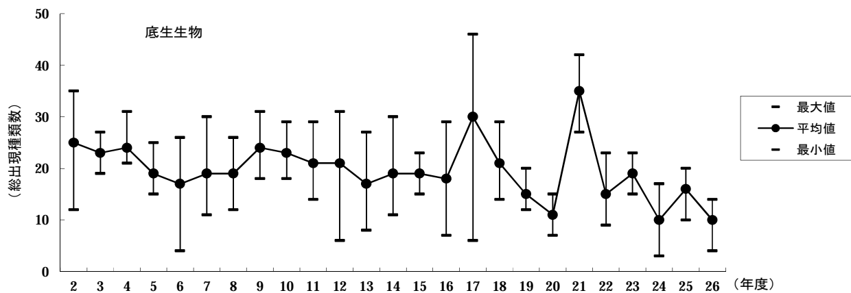
図 3-2-12 海生生物の総出現種数の経年変化
