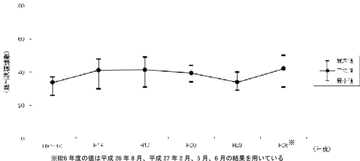
図 3-1-8 陸域生態系（鳥類）の総出現種類数の経年変化
