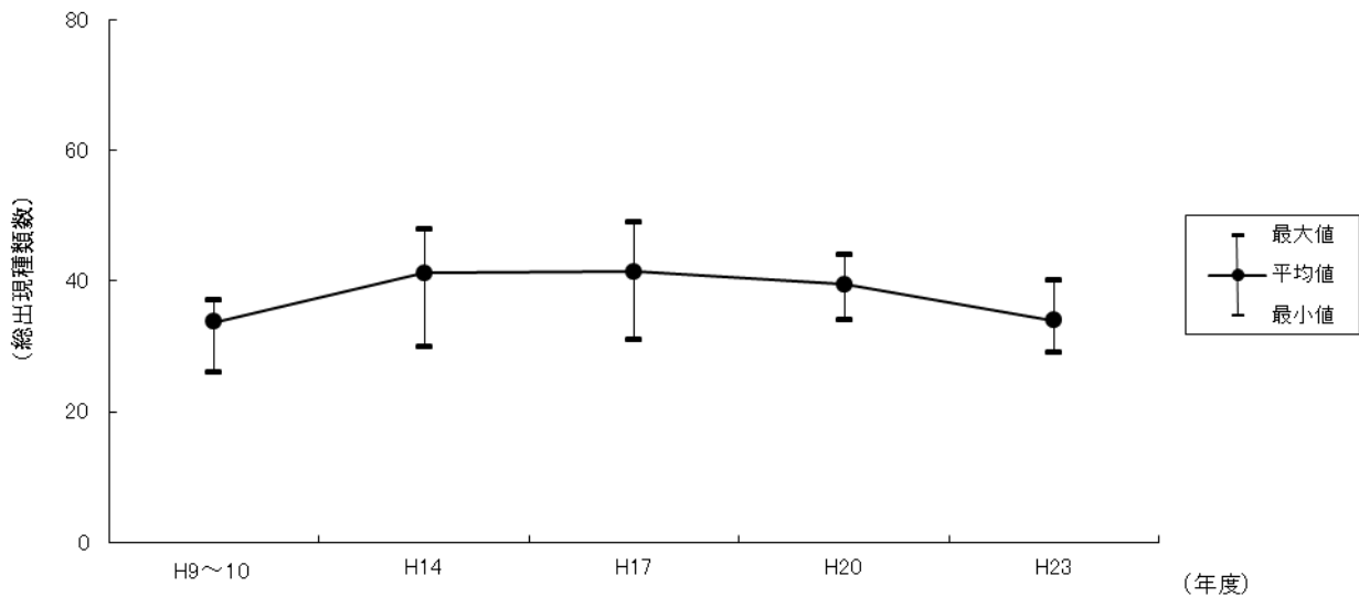
図 3-4-7 陸域生態系（鳥類）の総出現種類数の経年変化
