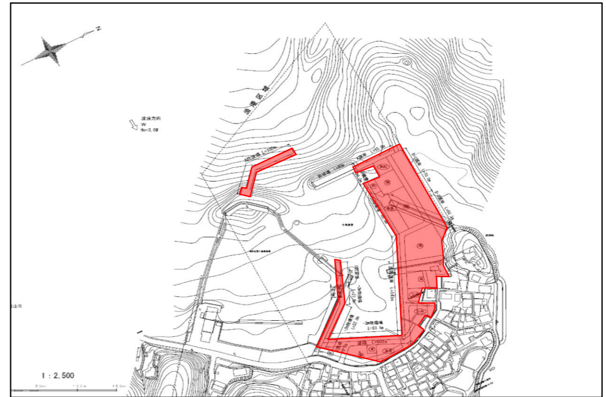
① -2m物揚場
