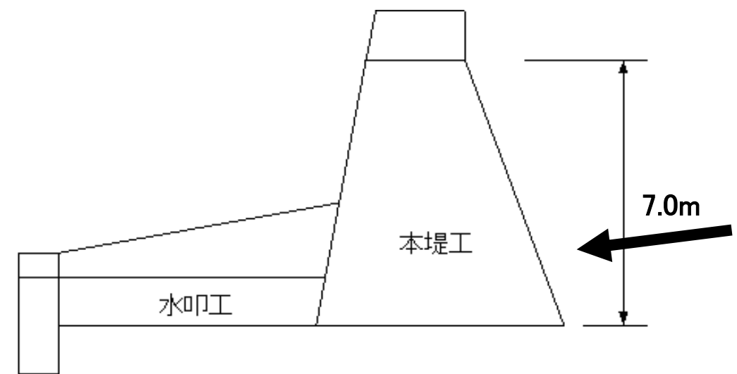
標準断面図
