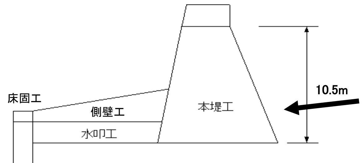
標準断面図
