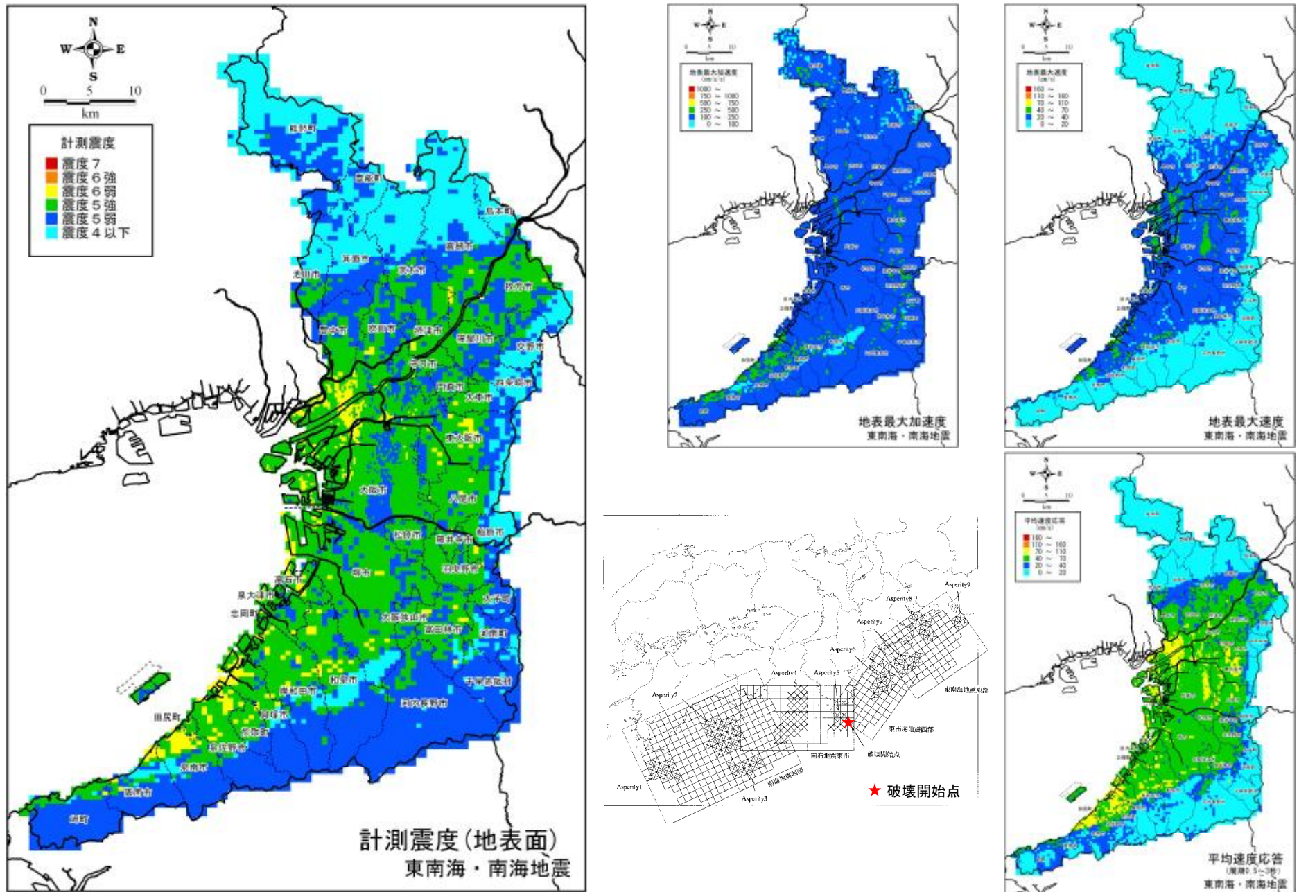
図 2-21 ステップ 3 の地震動予測結果 [東南海・南海地震]
