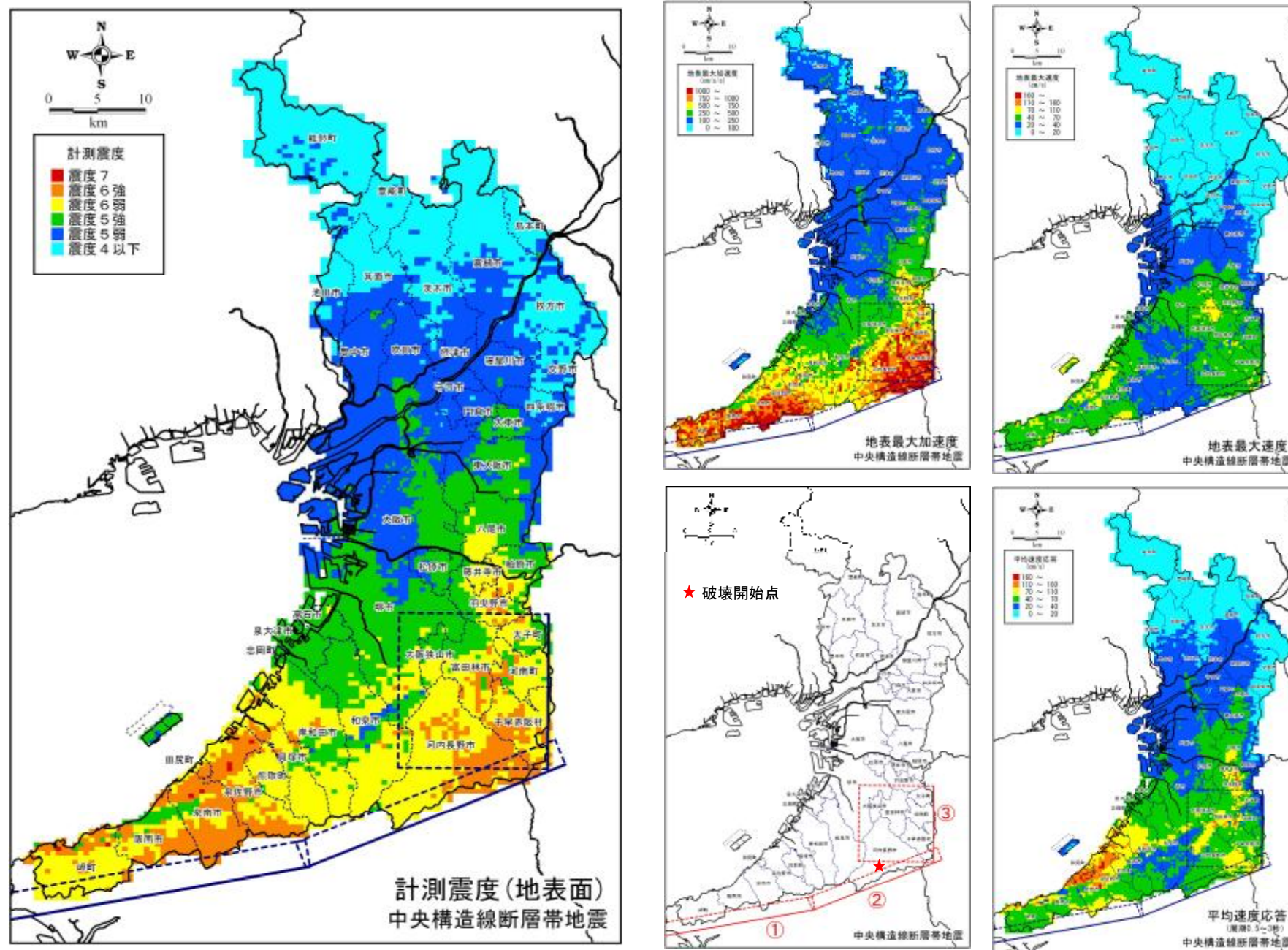
図 2-20 ステップ 3 の地震動予測結果〔中央構造線断層帯地震〕
