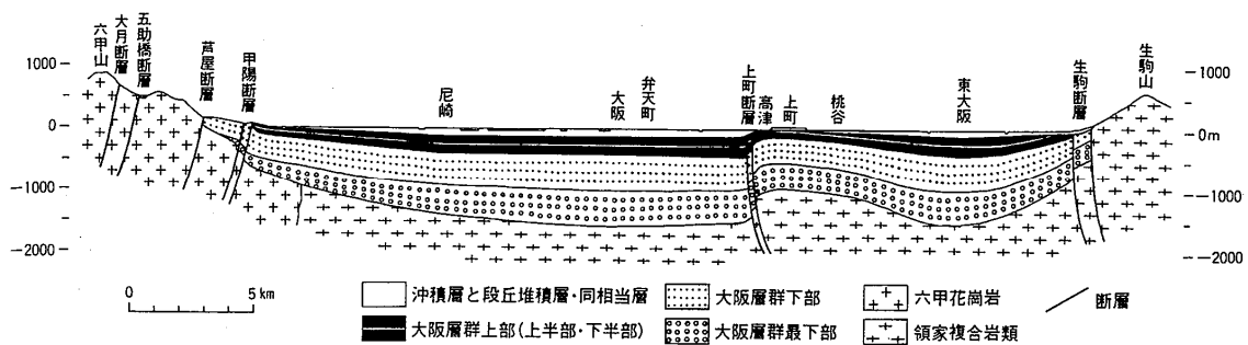
図 3-3 大阪堆積盆地の東西地質断面 (市原編, 1993)
