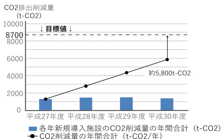
図-4：二酸化炭素削減量
