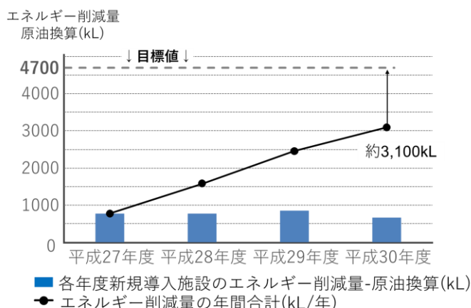
図-3：エネルギー削減量
