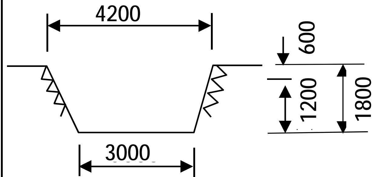
標準断面図
