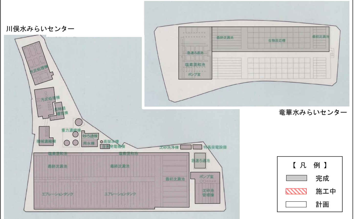
川俣水みらいセンター、竜華水みらいセンター(処理場)
