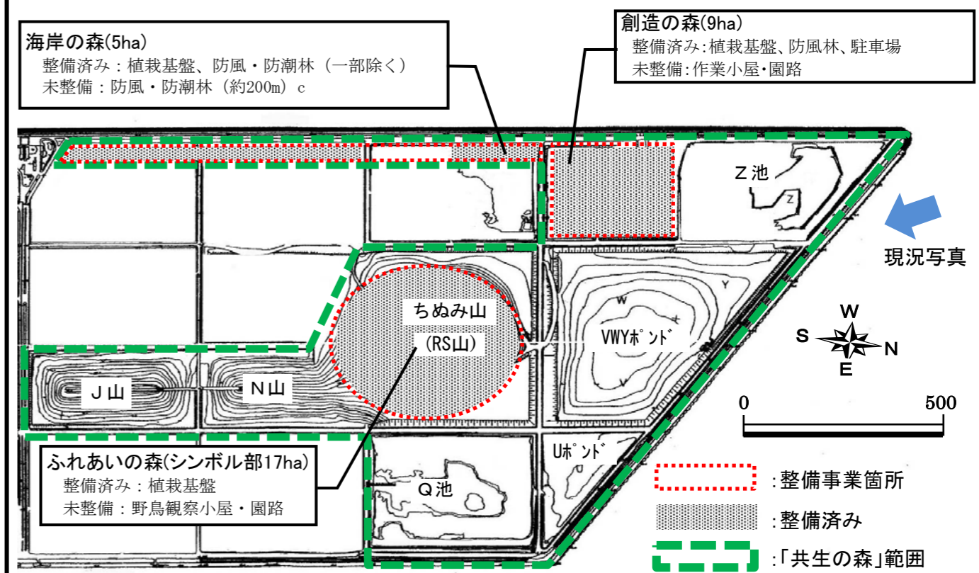
平面図
