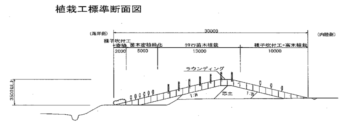
標準断面図
