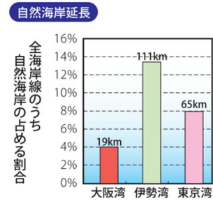
閉鎖性海域における浅場・干潟・自然海岸の比較 (出典：大阪湾再生行動計画パンフレット (2023 年度))
