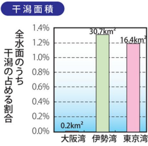
閉鎖性海域における浅場・干潟・自然海岸の比較 (出典：大阪湾再生行動計画パンフレット (2023 年度))
