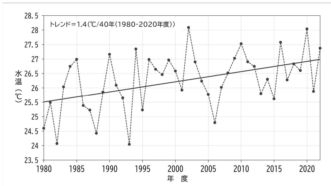
大阪湾（※）における夏季（7～9月）の水温変化
