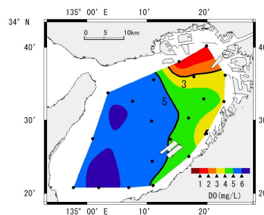
夏基底層 DO の分布図 (2018～2020 年度平均)
