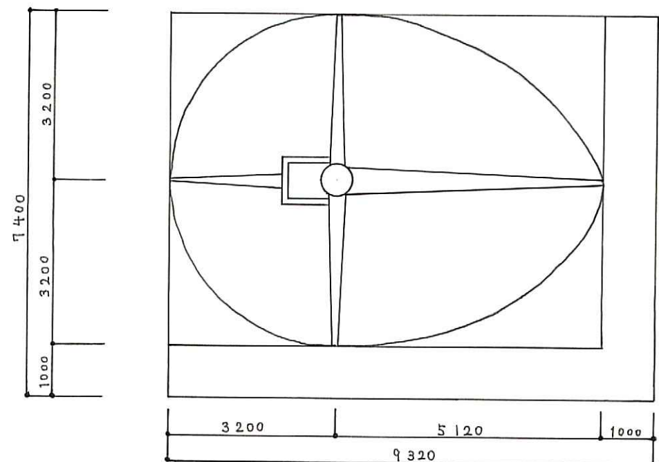
平面図 S1:100
