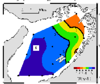
夏季底層DOの分布(2014～2016年度平均) 【出典】(地独)大阪府立環境農林水産総合研究所
