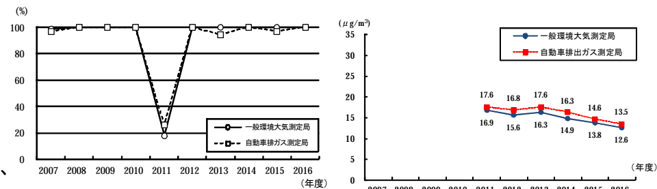
浮遊粒子状物質の環境保全目標達成率の推移
