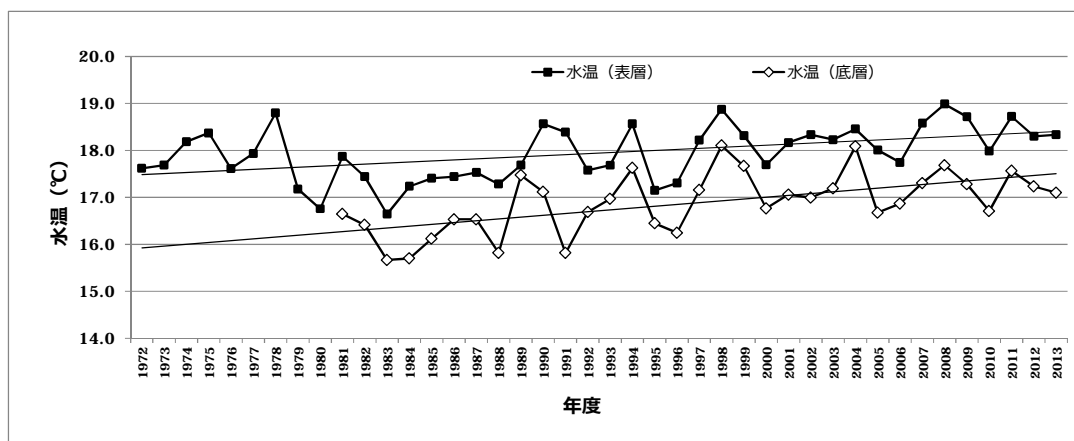
図 15- 2 水温の推移 (B 類型海域)
