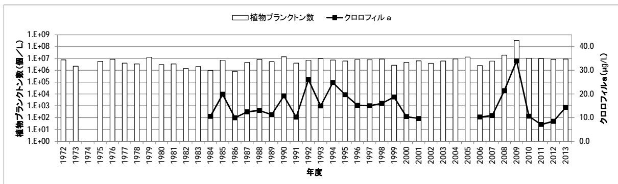
図 20-3 植物プランクトン数及びクロロフィル a の推移 (C 類型海域) (大阪府が測定する環境基準点におけるデータ)
