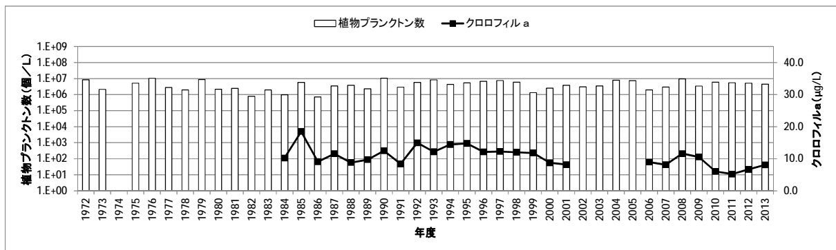
図 20-2 植物プランクトン数及びクロロフィル a の推移 (B 類型海域) (大阪府が測定する環境基準点におけるデータ)
