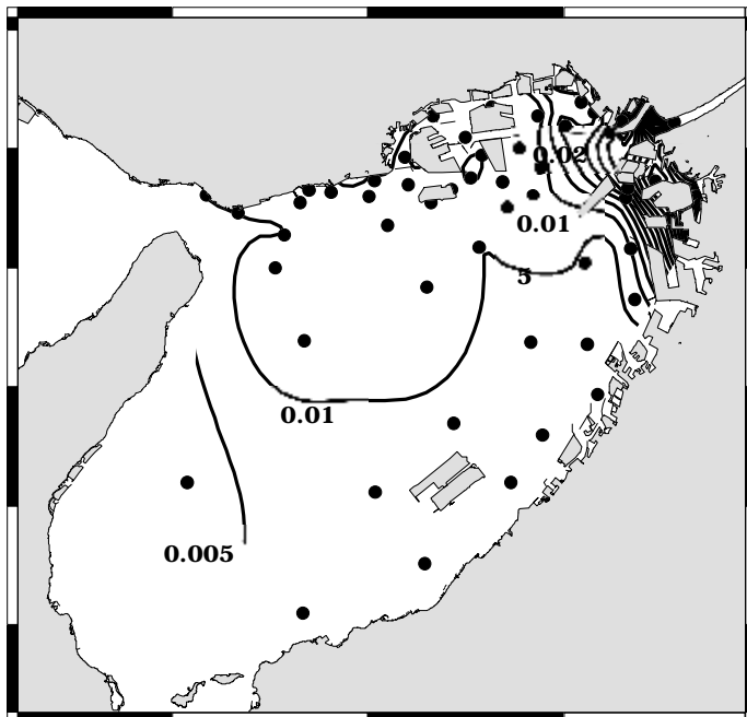
図5 DIP (表層、コンター間隔 : 0.005mg/L)
