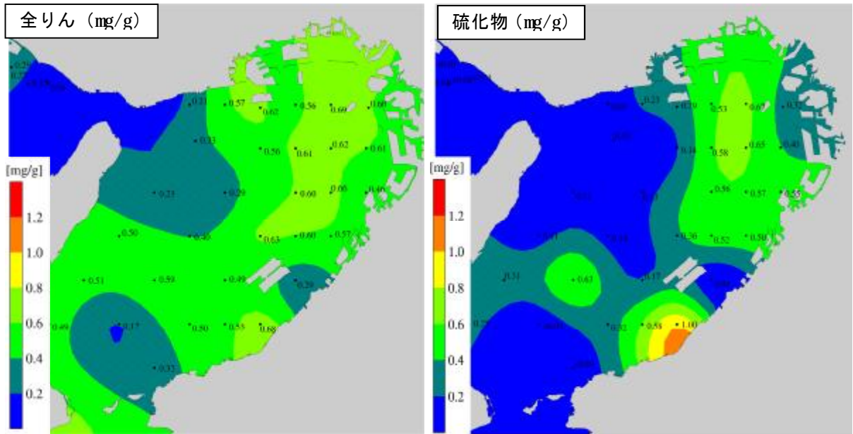
図8 底質の水平分布（2）（平成27年度 瀬戸内海環境情報基本調査）
