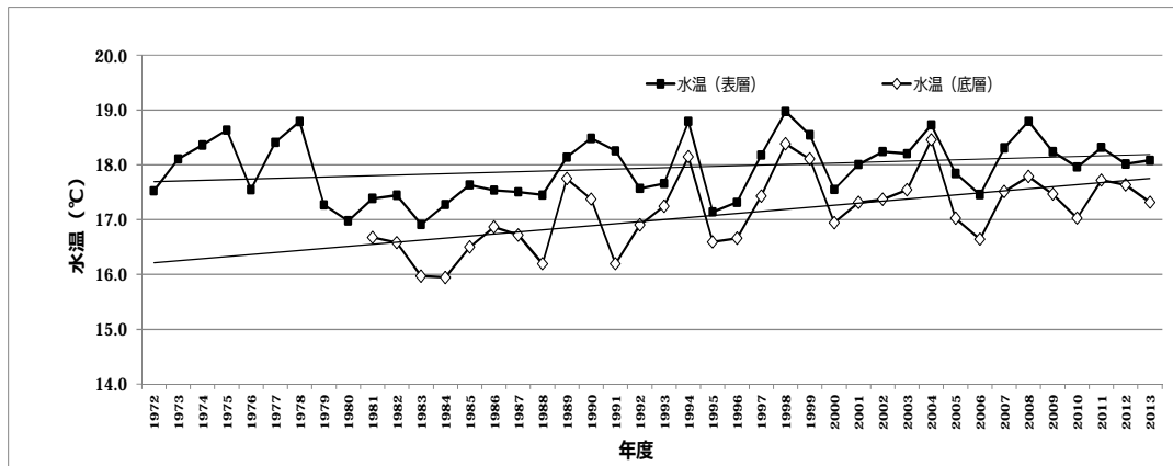
図 15- 1 水温の推移 (A 類型海域)
