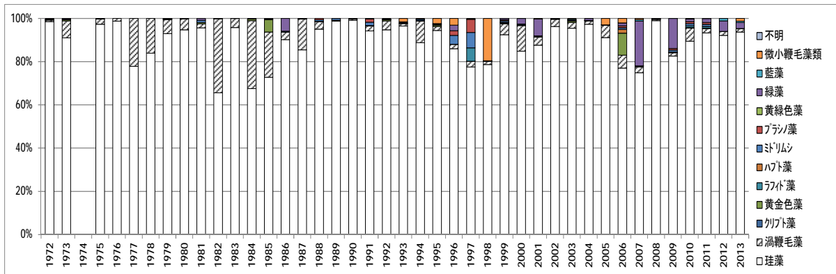
図 21-1 植物プランクトンの綱別構成割合の推移 (A 類型海域) (大阪府が測定する環境基準点におけるデータ)
