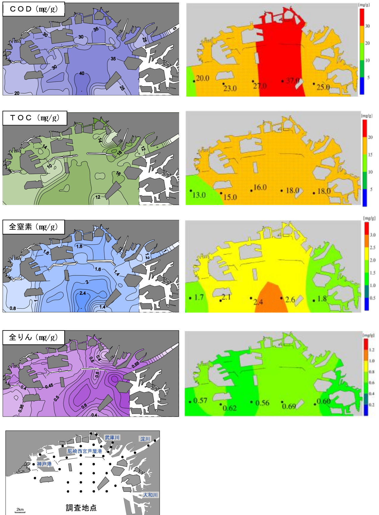
図 14 湾奥部での底質調査結果 (2)
