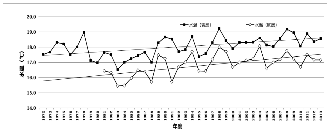
図 15- 3 水温の推移 (C 類型海域)
