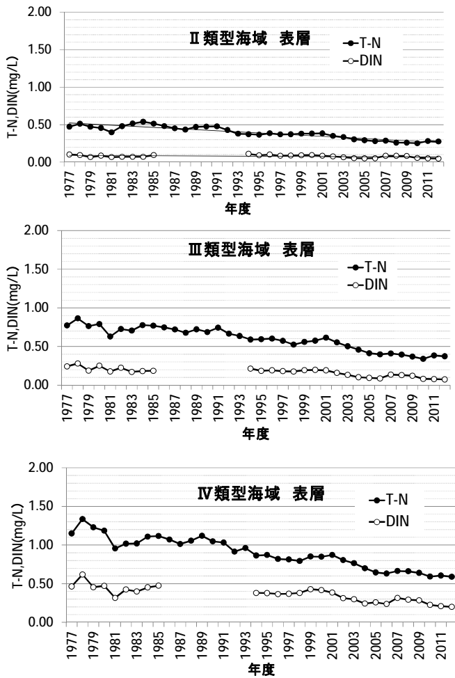
図 11 表層の全窒素(T-N)及び溶存性無機態窒素(DIN)の年平均値(mg/L)の経年変化(大阪府が測定する環境基準点におけるデータ)
