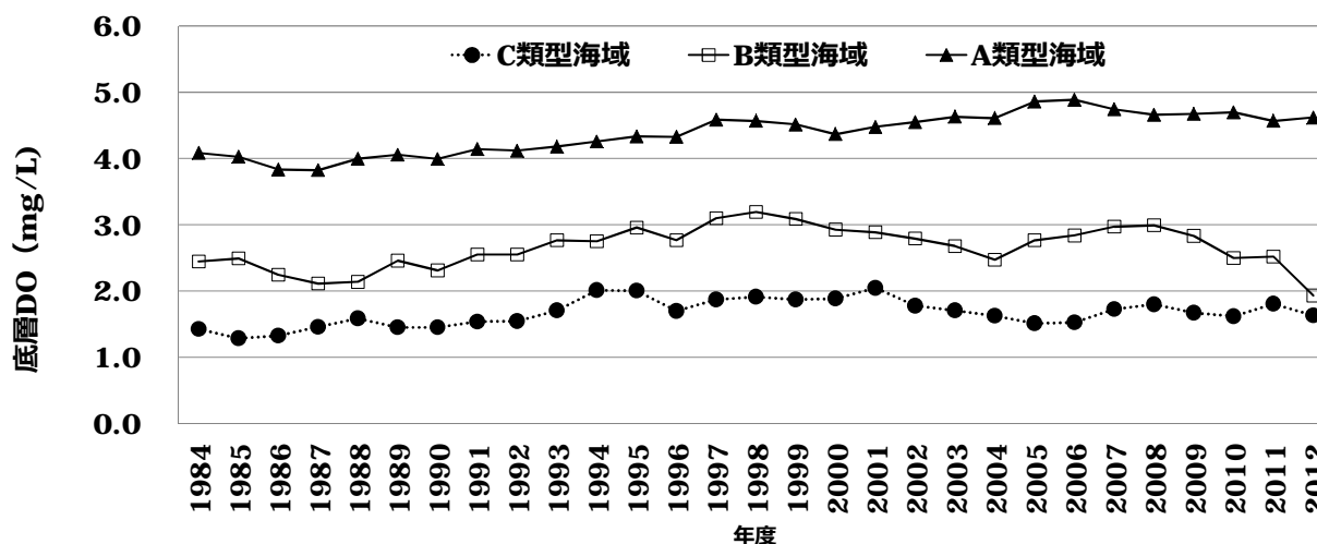
図 17 底層 DO の年度最小値 (mg/L) の経年変化 (大阪府が測定する環境基準点におけるデータ。年度につき 1 個のデータであり、年々の変動が大きいため、5 年移動平均して経年的な変化傾向を見やすくしている。)
