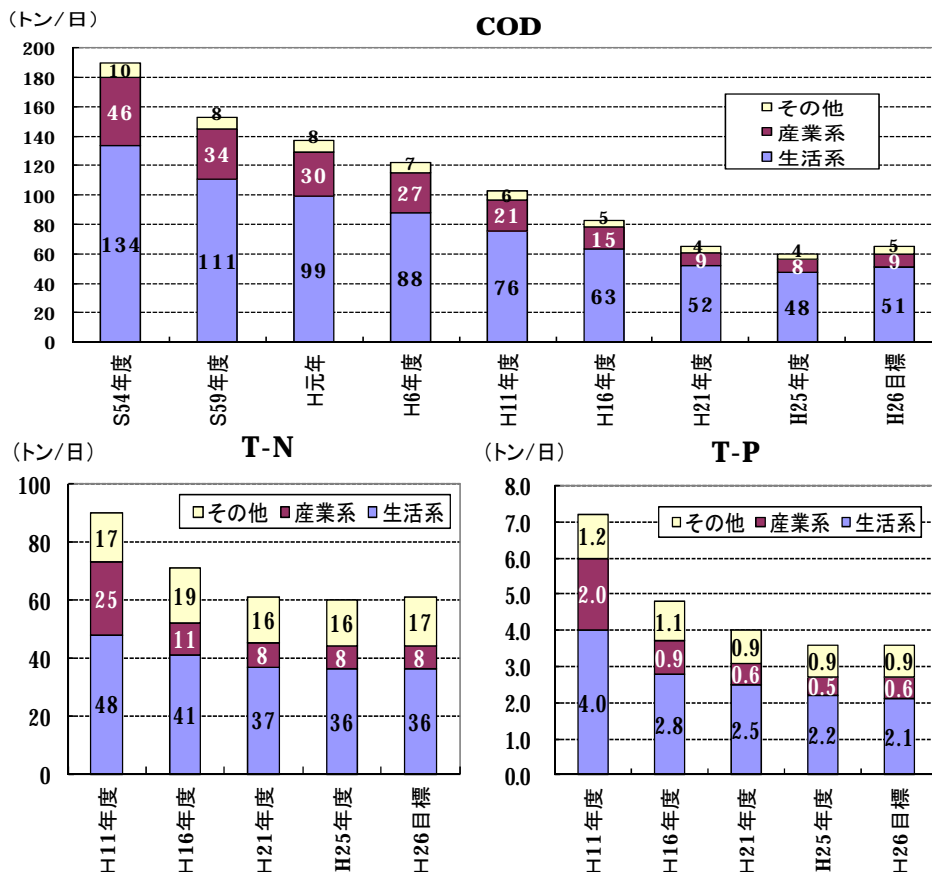
図30 COD、窒素、りに係る汚濁負荷量の推移
