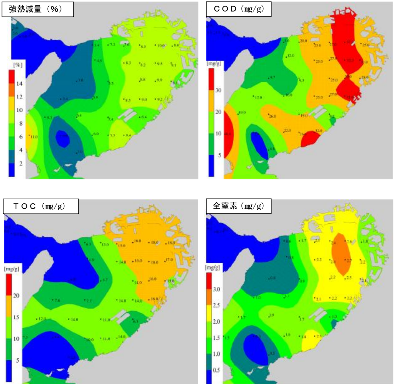
図 8 底質の水平分布 (1) (平成 27 年度 瀬戸内海環境情報基本調査)
