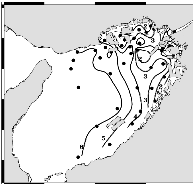
図7 8月の底層DO (コンター間隔：1 \text{mg/L} )
