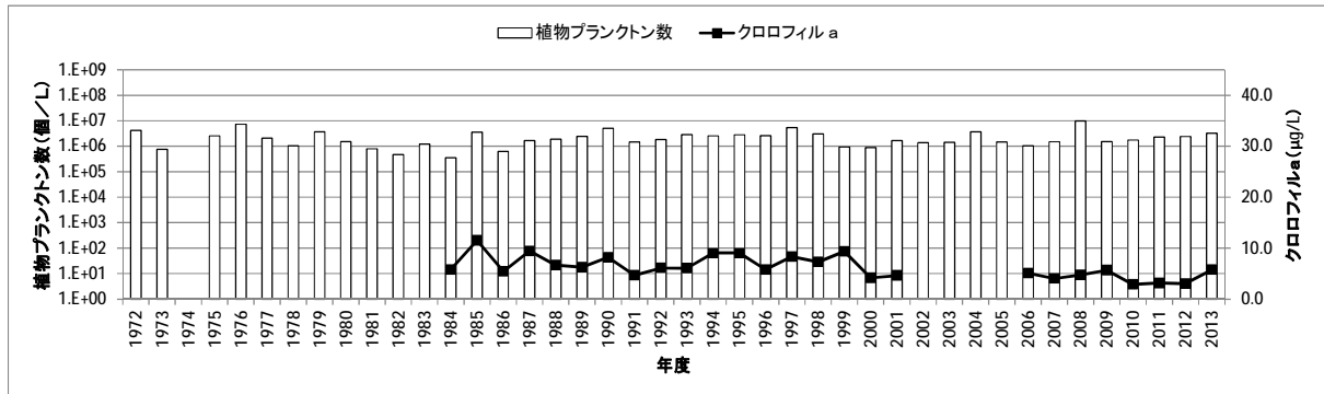
図 20-1 植物プランクトン数及びクロロフィル a の推移 (A 類型海域) (大阪府が測定する環境基準点におけるデータ)
