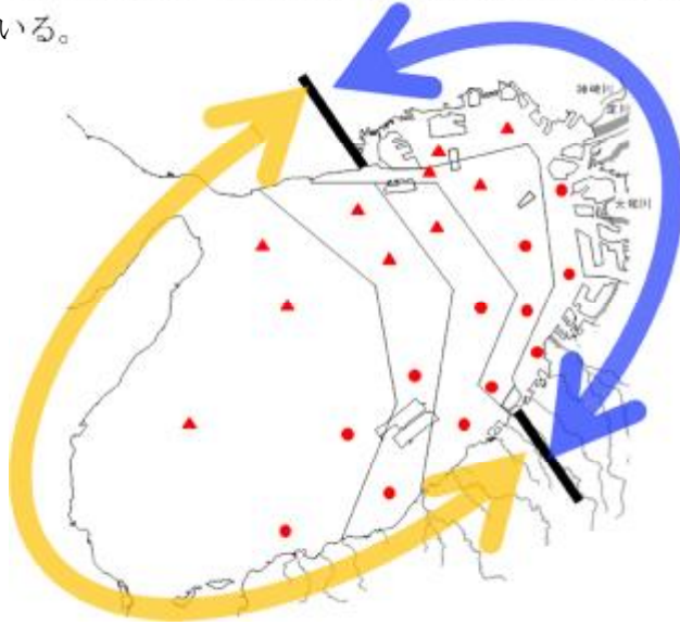
図20 図12～図14の重ね合わせ
