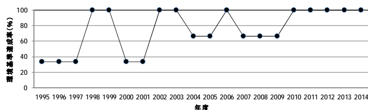
図9-2 全りんの環境基準達成率の推移
