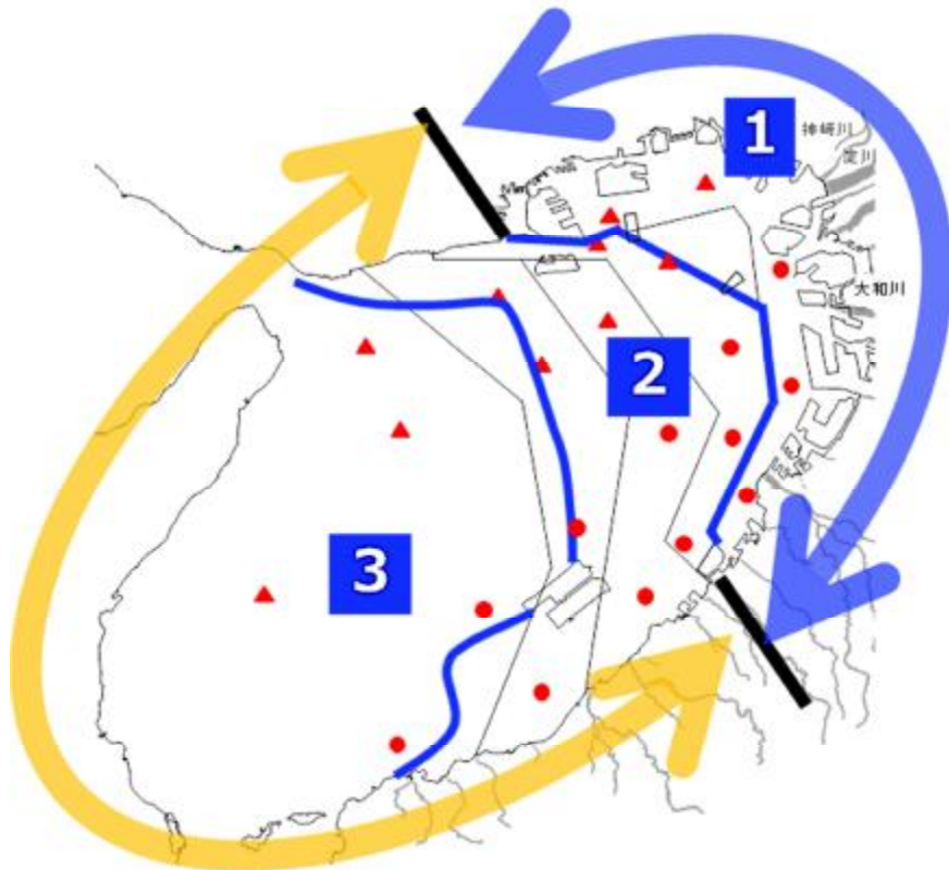
図21 大阪湾のゾーニング
