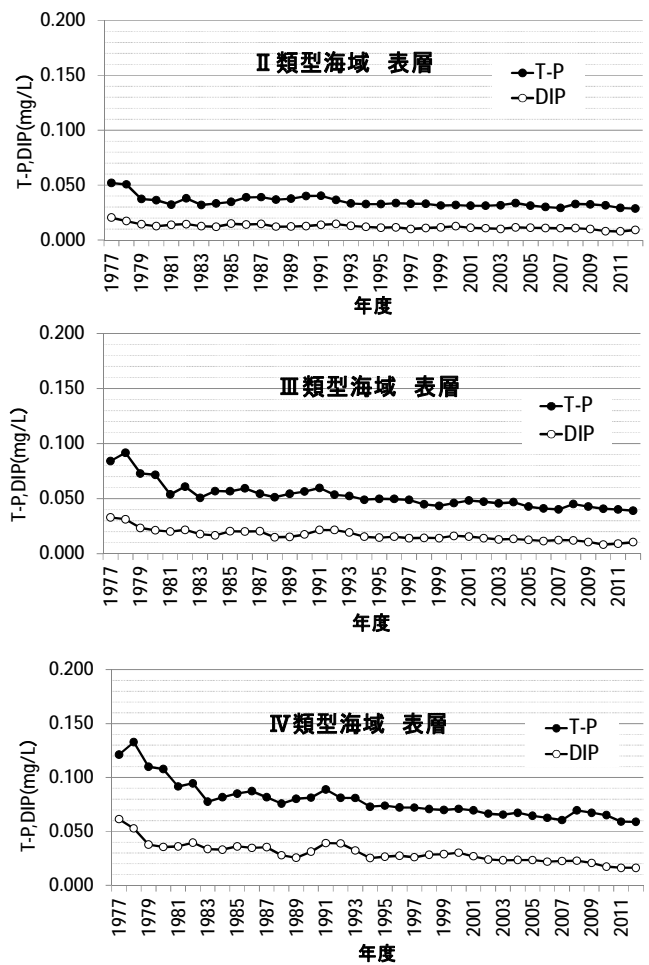
図 12 表層の全りん(T-P)及び溶存性無機態りん(DIP)の年平均値(mg/L)の経年変化(大阪府が測定する環境基準点におけるデータ)
