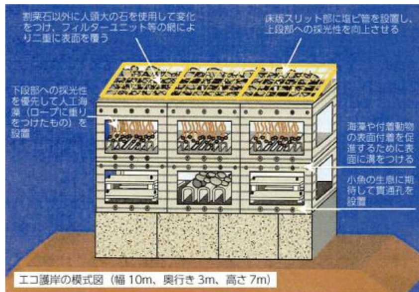
図 29 泉大津沖処分場のエコ護岸
