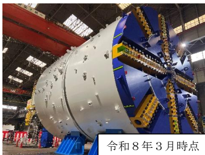
写真1：鶴見調節池 (シールドマシン)
