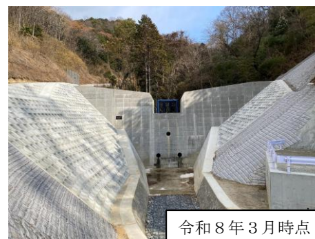
写真5：北川支川砂防堰堤
