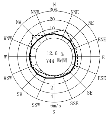
風配図 [令和5年10月分]
