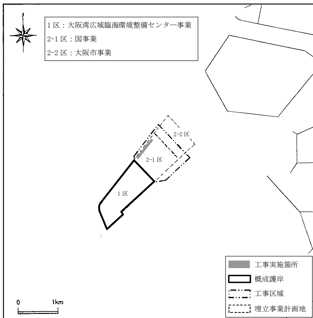
図-2 工事の実施状況（平成26年2月）
