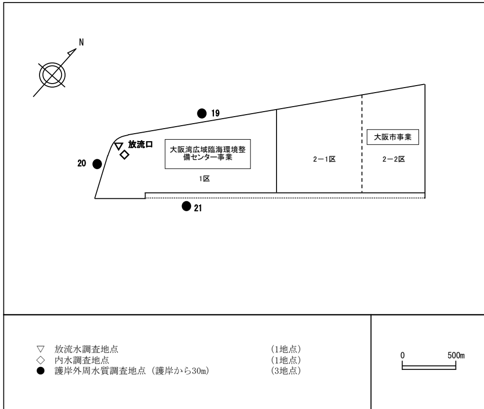
図－1 廃棄物処分場周辺における水質(健康項目等)の調査地点(平成26年11月)
