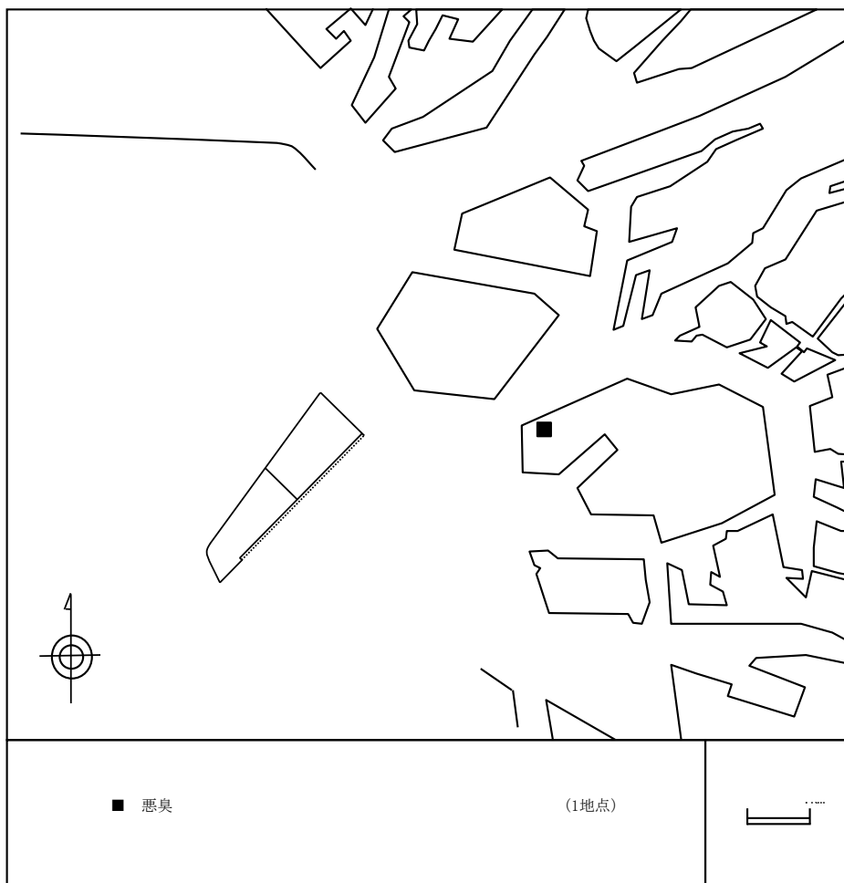
図-1 悪臭の調査地点(平成 26 年 9 月)
