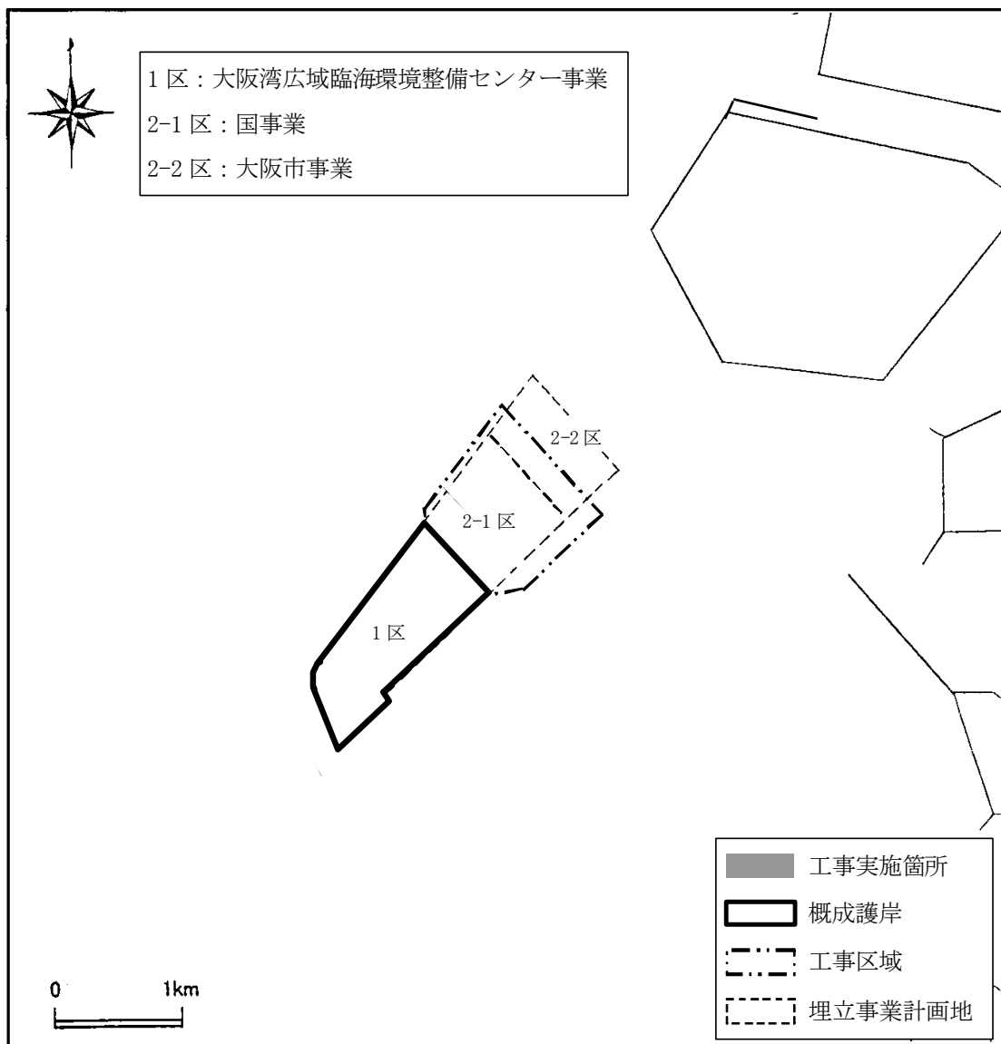
図-2 工事の実施状況（平成27年11月）
