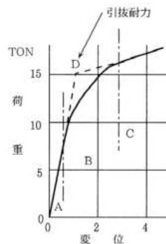
図-1 ロックボルト引抜試験
