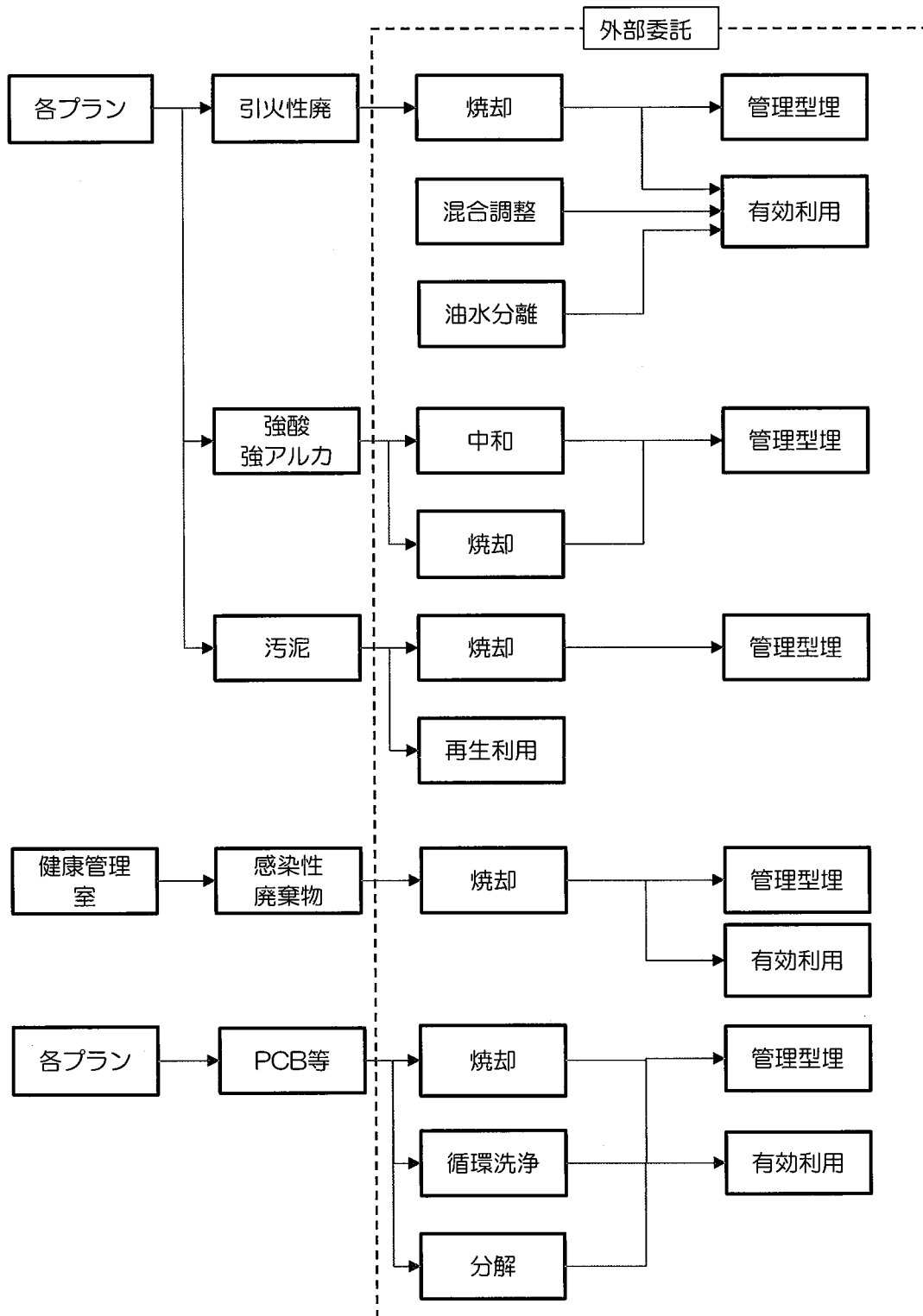
特別管理産業廃棄物処理工程図
