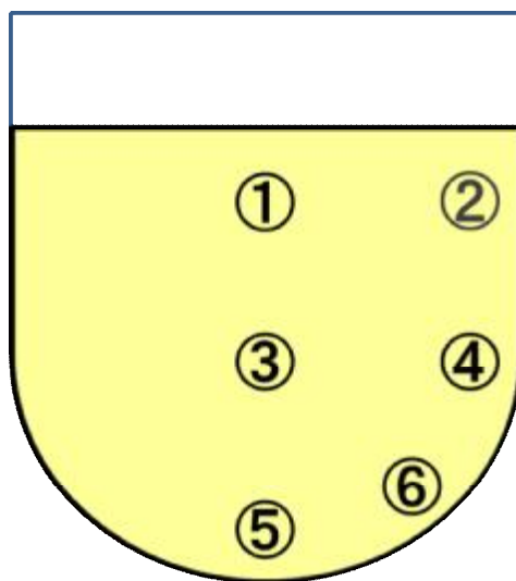
図2 練合機からの検体採取箇所
