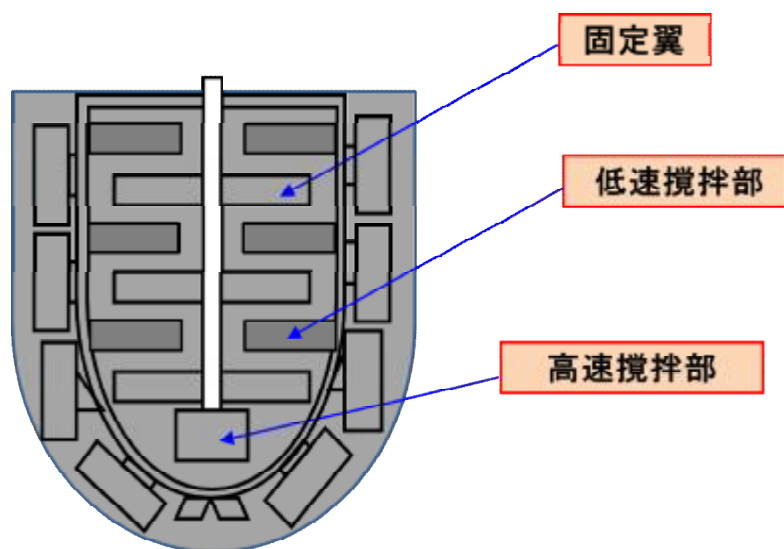
図1 練合機（攪拌槽）の概略図例
