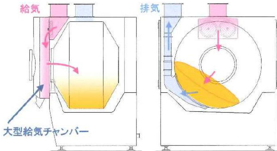
【通気式コーティング装置の例】
