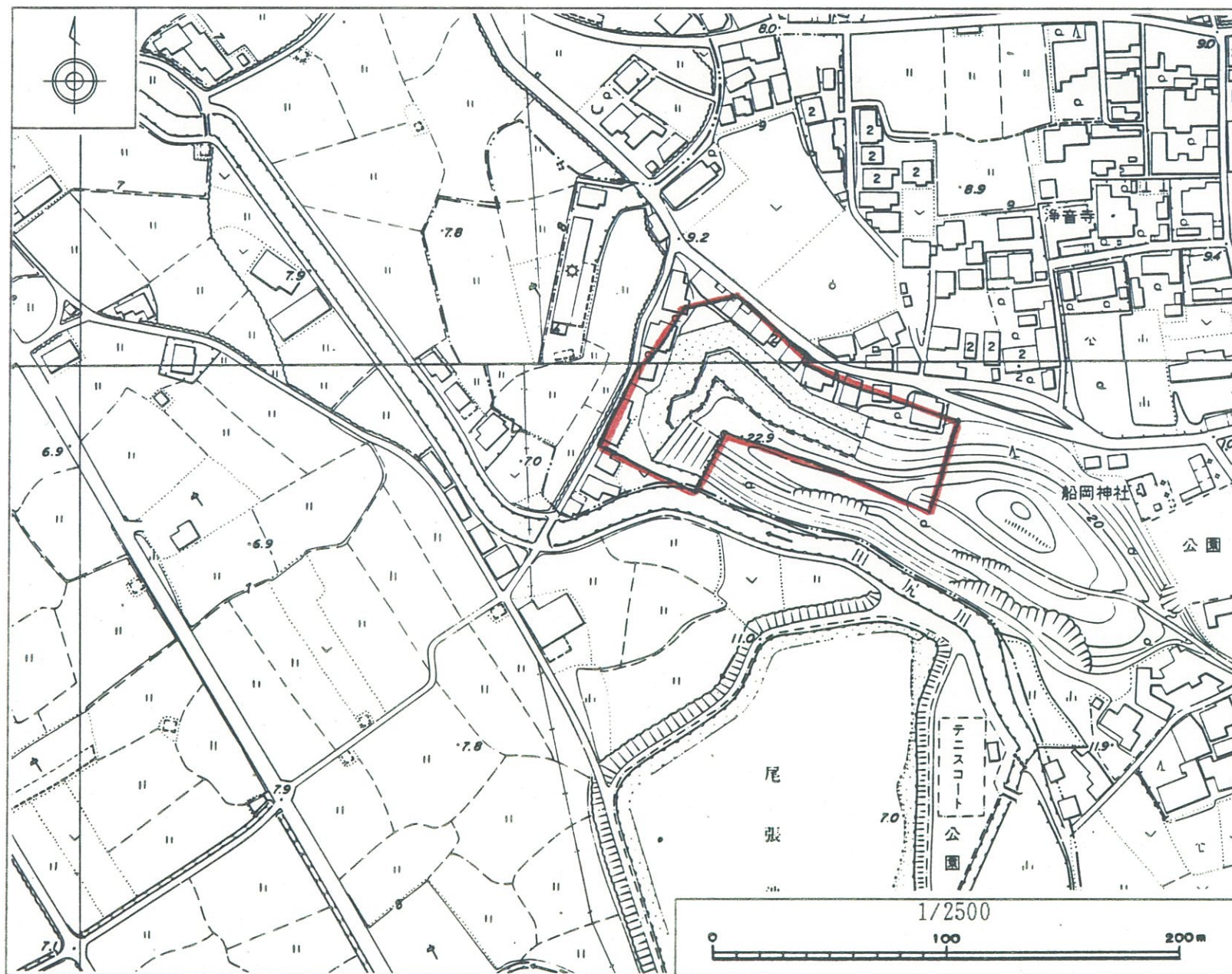
平面図
