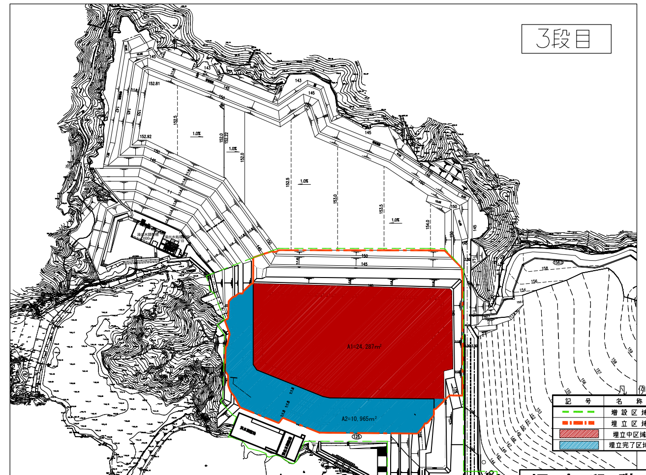
埋立段階図 1
