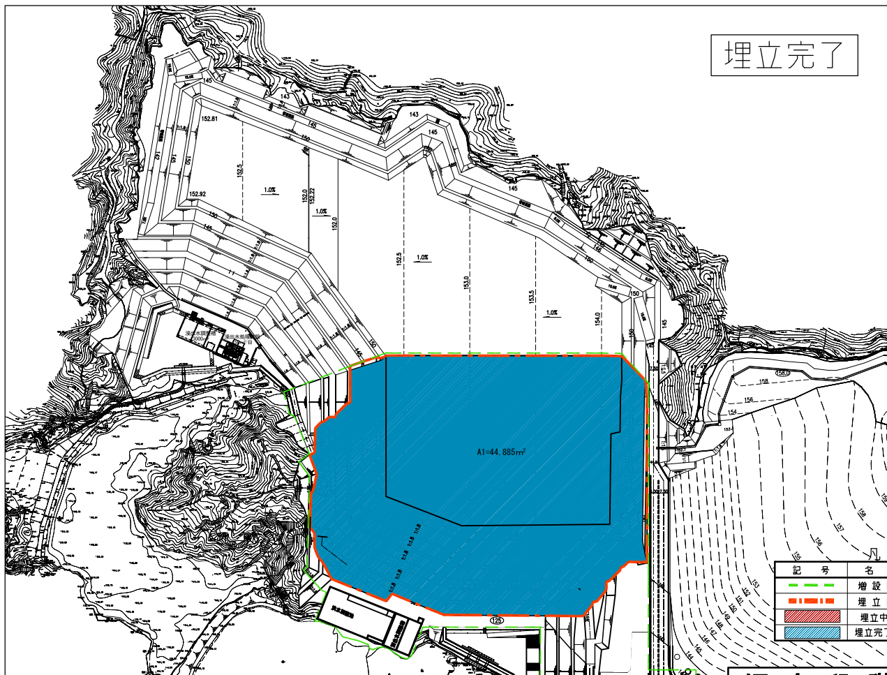
埋立段階図 2
