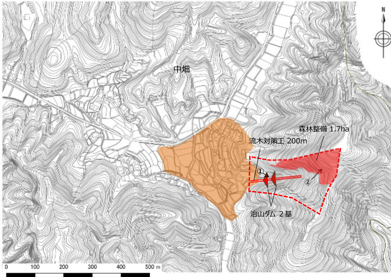
【平面図】
