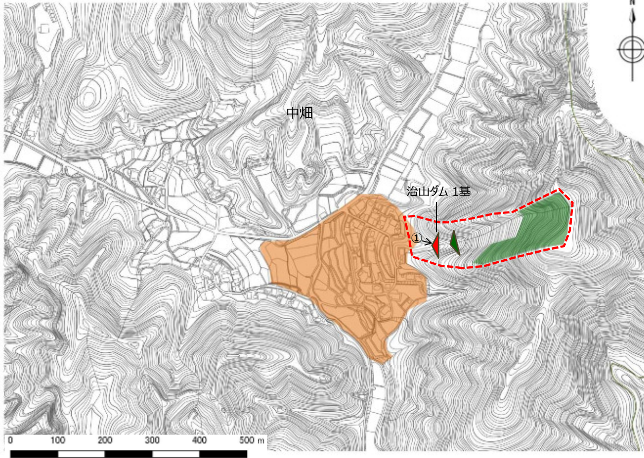
【平面図】
