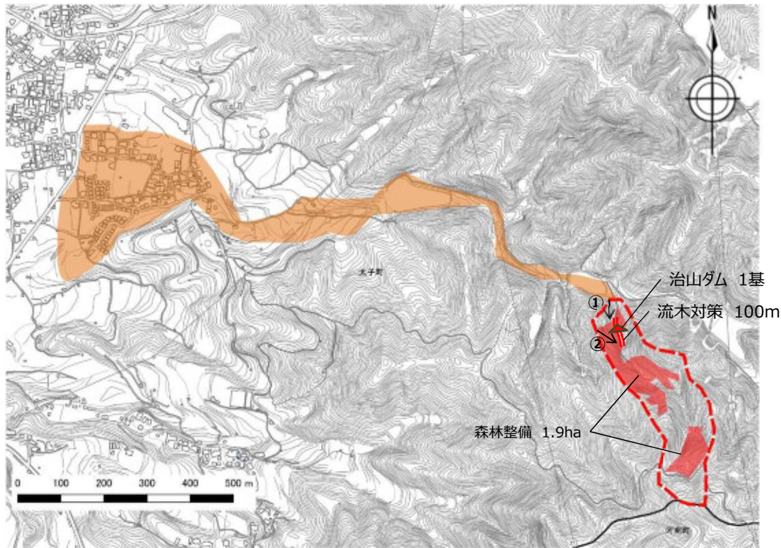
【平面図】
