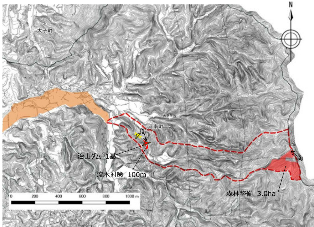
【平面図】
