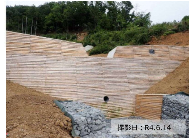
写真① 治山ダム（コンクリート）の設置状況
