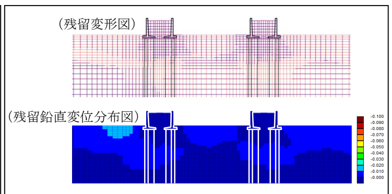
図3-14 点検結果（橋軸直角方向）
