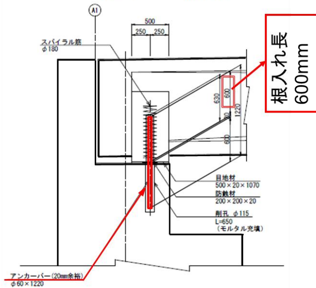
アンカーバー詳細図
