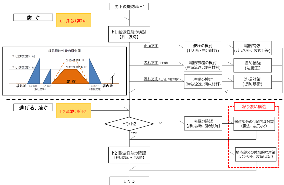
図2-12 検討フロー
