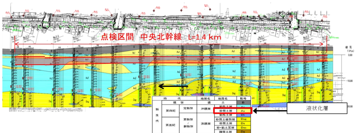
図3-20 液状化判定
