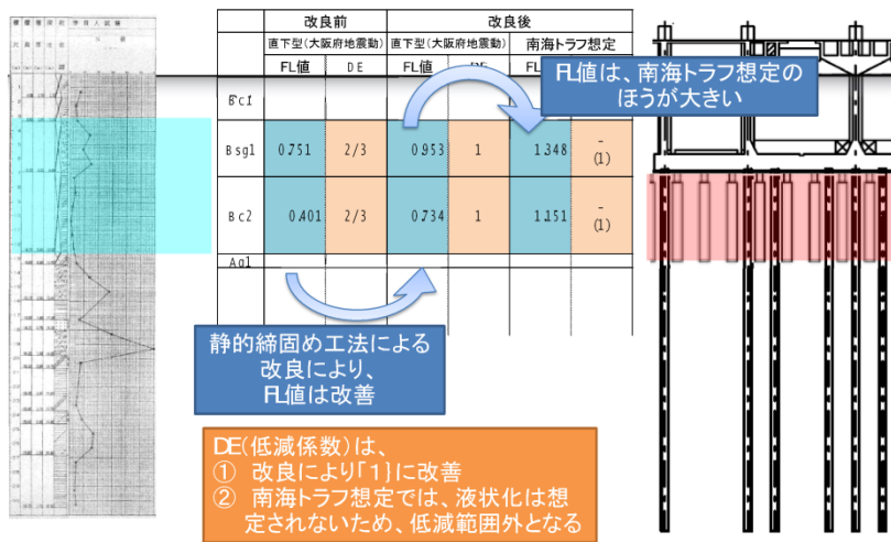
図3-17 北部水みらいセンター液状化判定
