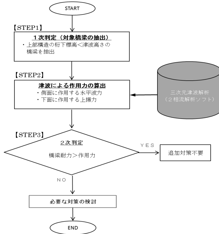
図2-14 点検フロー
