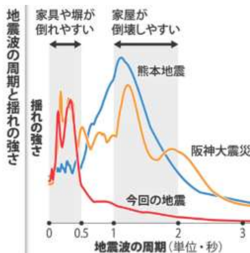
図表-1 地震波の周期と揺れの強さ
