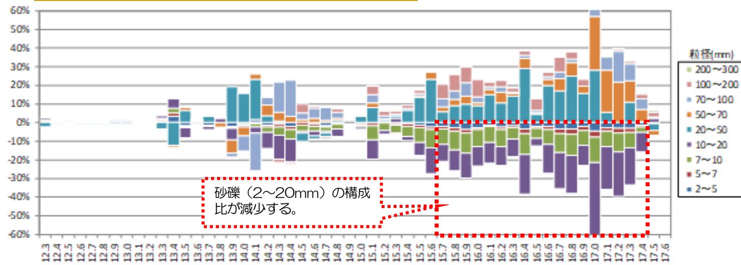
図 2-7 安威川河床材料の粒度組成の変化 (ダムがある場合とダムがない場合の河床材料の差分)
