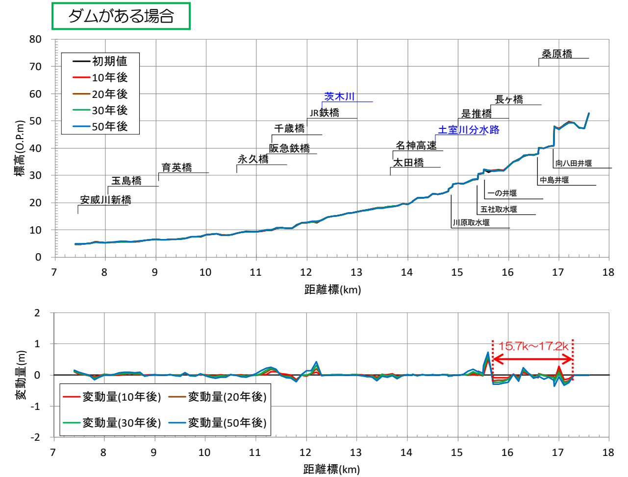
図 2-3 安威川河床変動解析結果（ダムがある場合）
