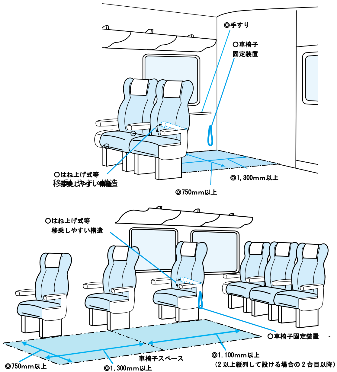
参考 4-1-42：車椅子スペースの例
