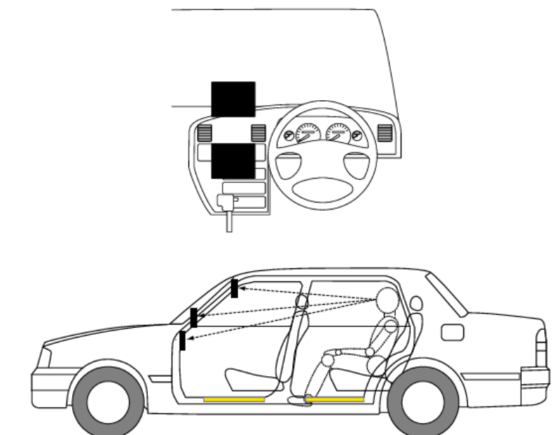
参考 4-3-18：タクシーメーターの位置の例
