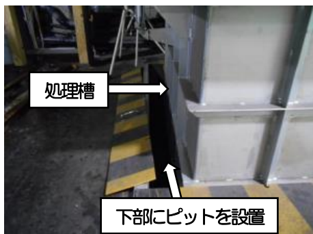
処理槽の下部にピットを設置
