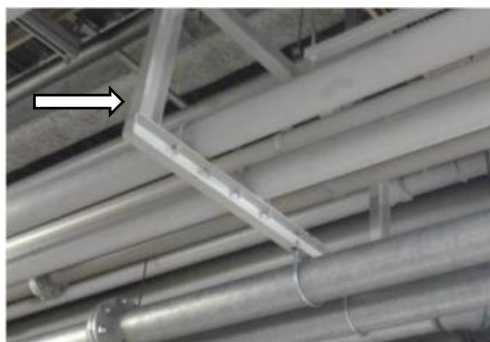
配管の吊り金具の補強
