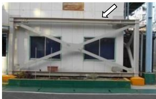
ブレース（建屋外）
