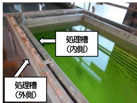
処理槽を二重に設置
