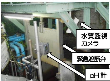
pH計、監視カメラ、緊急遮断弁
