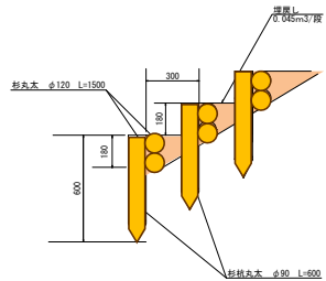
丸太階段工 断面図 S=1/1.0
