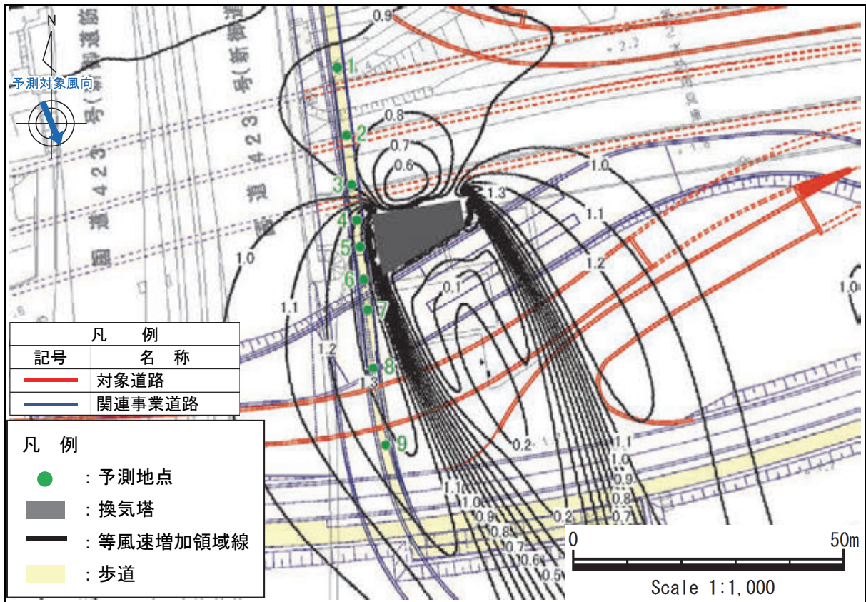
図 8-2-8(16) (仮称) 豊崎換気所 風速増加領域 (風向: 北北西)
