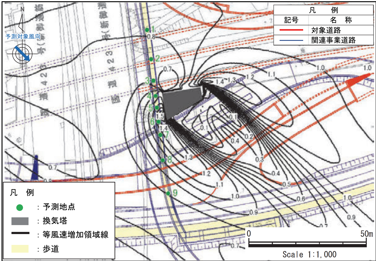
図 8-2-8(15) (仮称) 豊崎換気所 風速増加領域 (風向: 北西)
