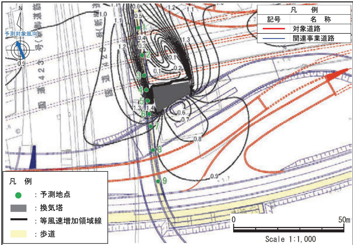
图 8-2-8(8) (仮称) 豊崎換気所 風速増加領域 (風向：南南東)
