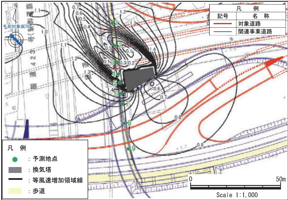
图 8-2-8(7) (仮称) 豊崎換気所 風速増加領域 (風向：南東)
