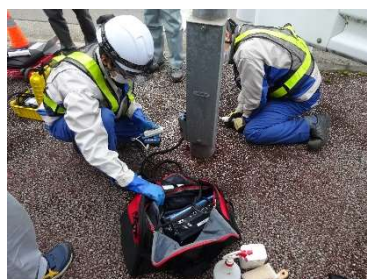
照明柱の非破壊調査
