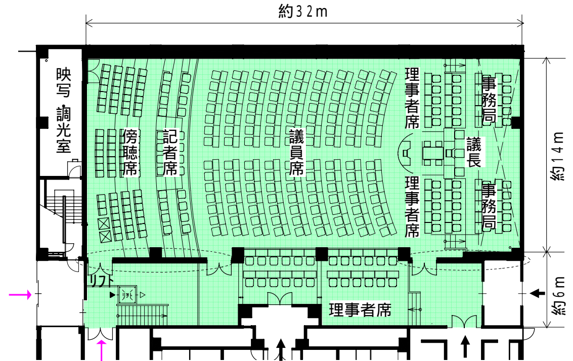
平面図
