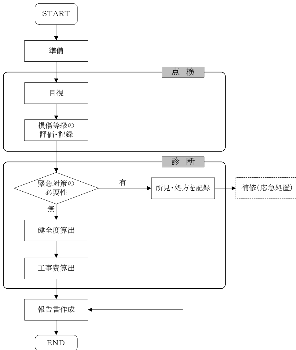
図5-1 点検の流れ
