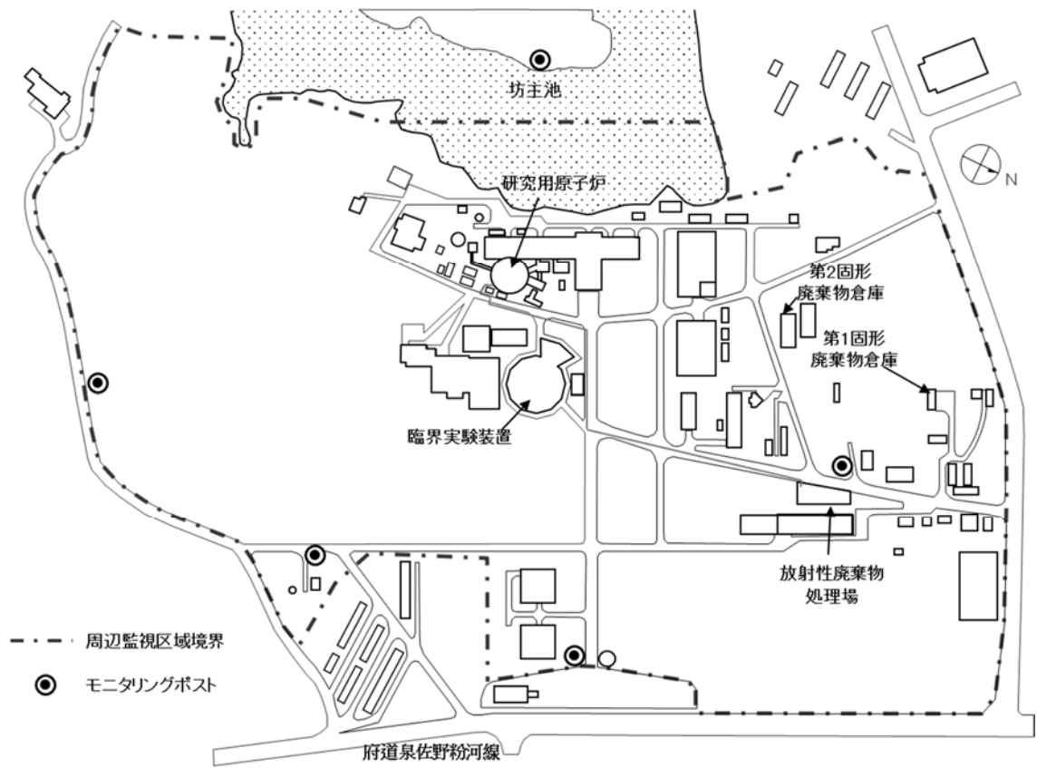
図1 敷地と主要な原子炉施設
