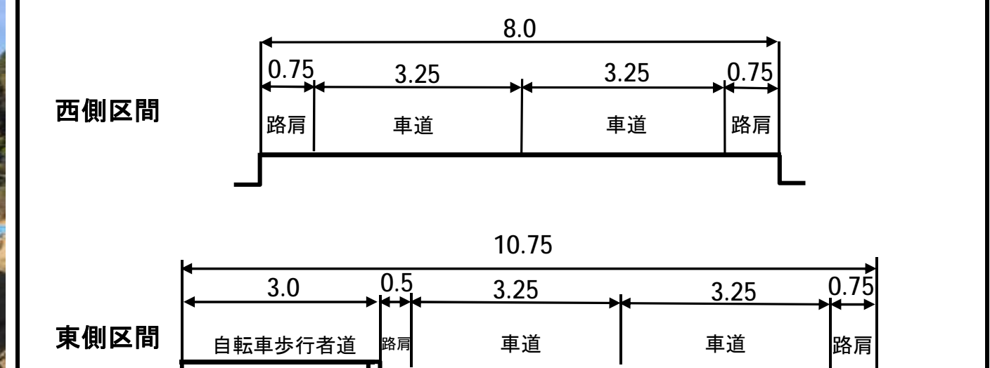
標準断面図 [単位:m]
