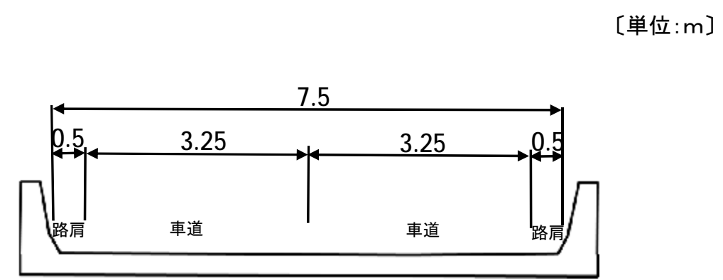
標準断面図
